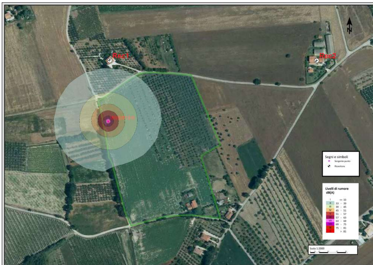
Figura 4 - Mappa del livello di rumore in emissione [dB(A)] su immagine satellitare
