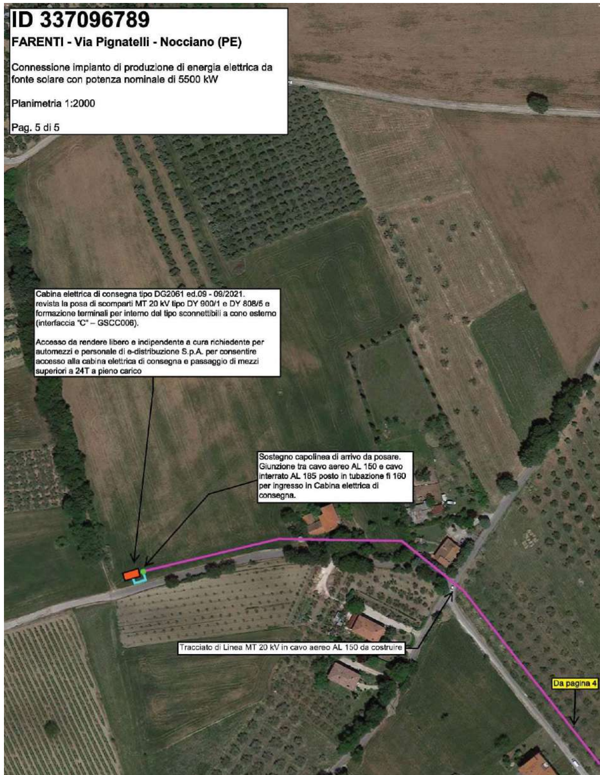
Figura 12 – PARTICOLARE SOLUZIONE DI CONNESSIONE – LATO CABINA UTENTE
