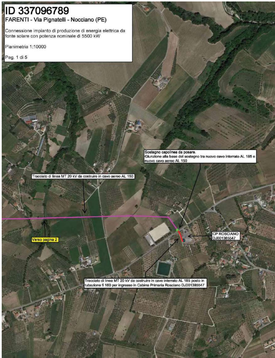
Figura 11 – PARTICOLARE SOLUZIONE DI CONNESSIONE – SU CP ROSCIANO
