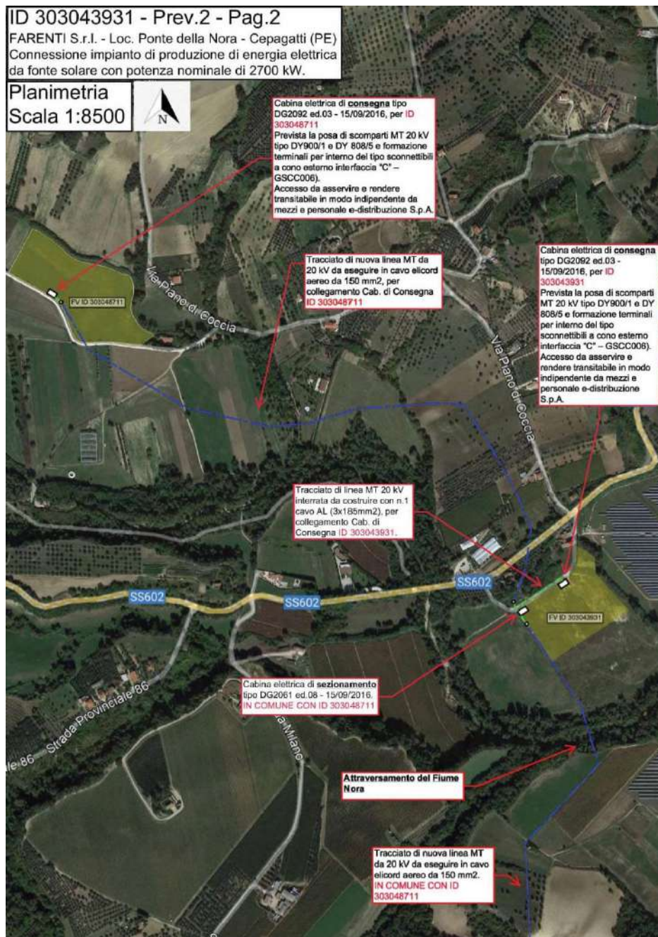
Figura 11 – PARTICOLARE SOLUZIONE DI CONNESSIONE – LATO NORD
