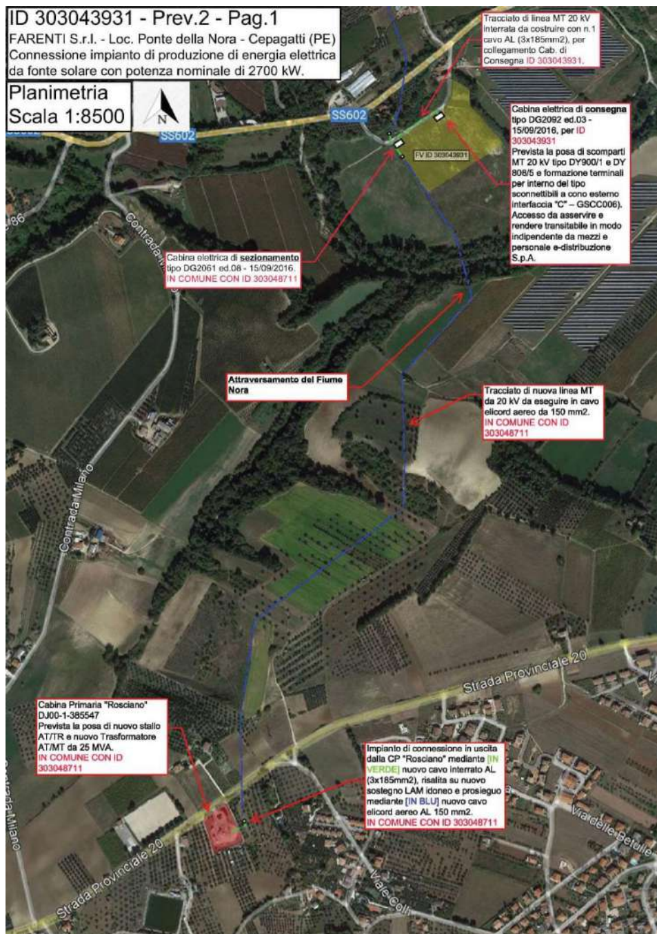
Figura 12 – PARTICOLARE SOLUZIONE DI CONNESSIONE – LATO SUD
