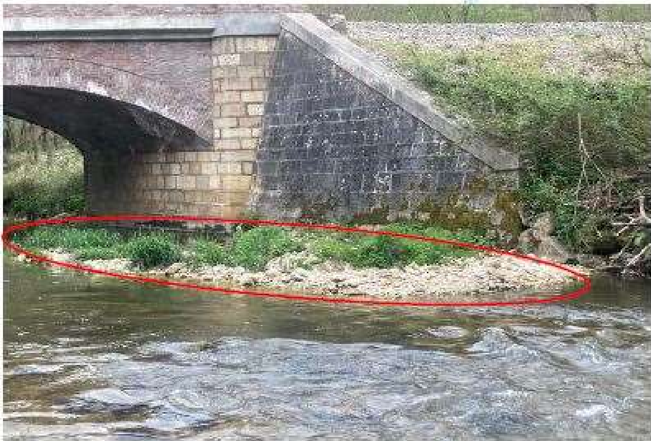
accumulo detritico al ponte 10
