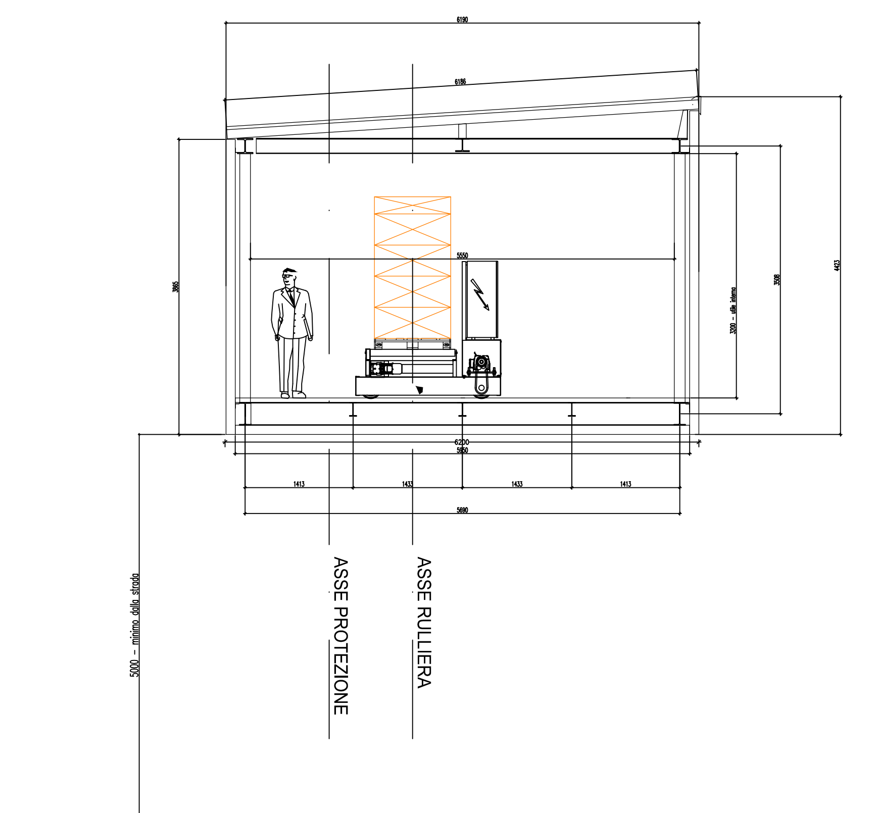
SEC. A-A Scala 1:50
