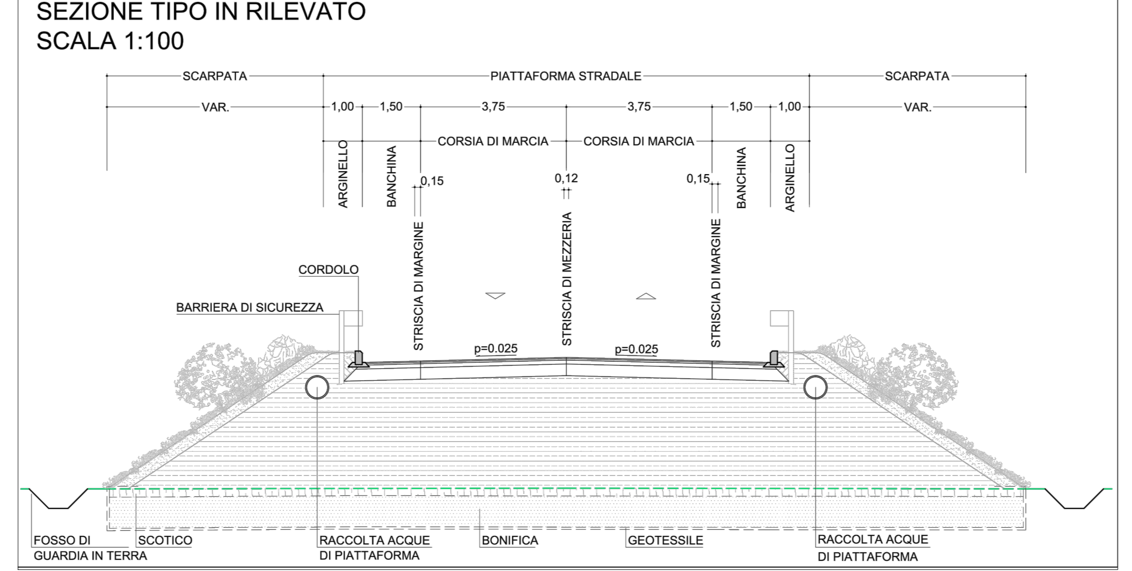
SEZIONE STRADALE TIPO PROPOSTA ANAS
