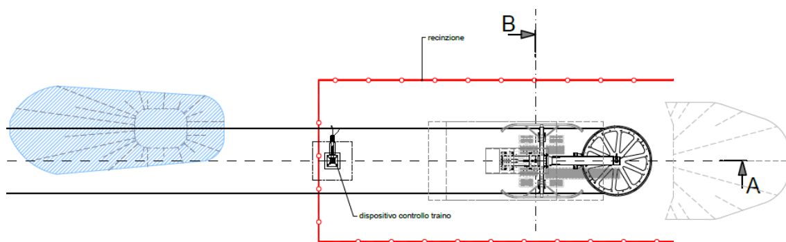
Fig. 17 – Pianta della stazione di monte in progetto.
