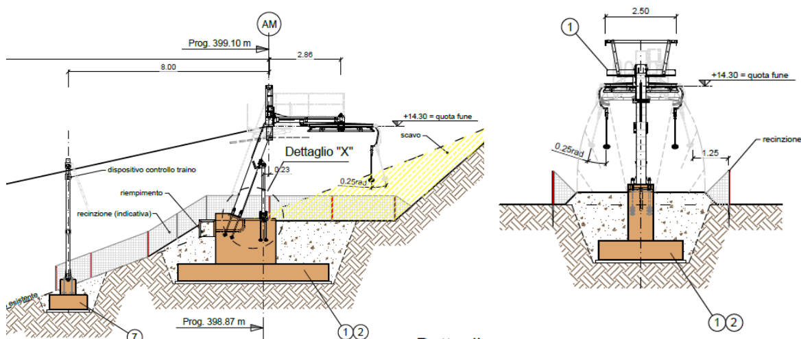
Fig. 18 – Profili stazione di monte in progetto.
