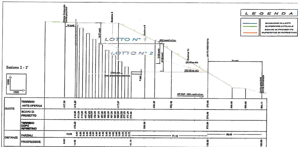
Fig. 14 – Sezione 2-2 di scavo (da Tav. I allegata allo SIA)
