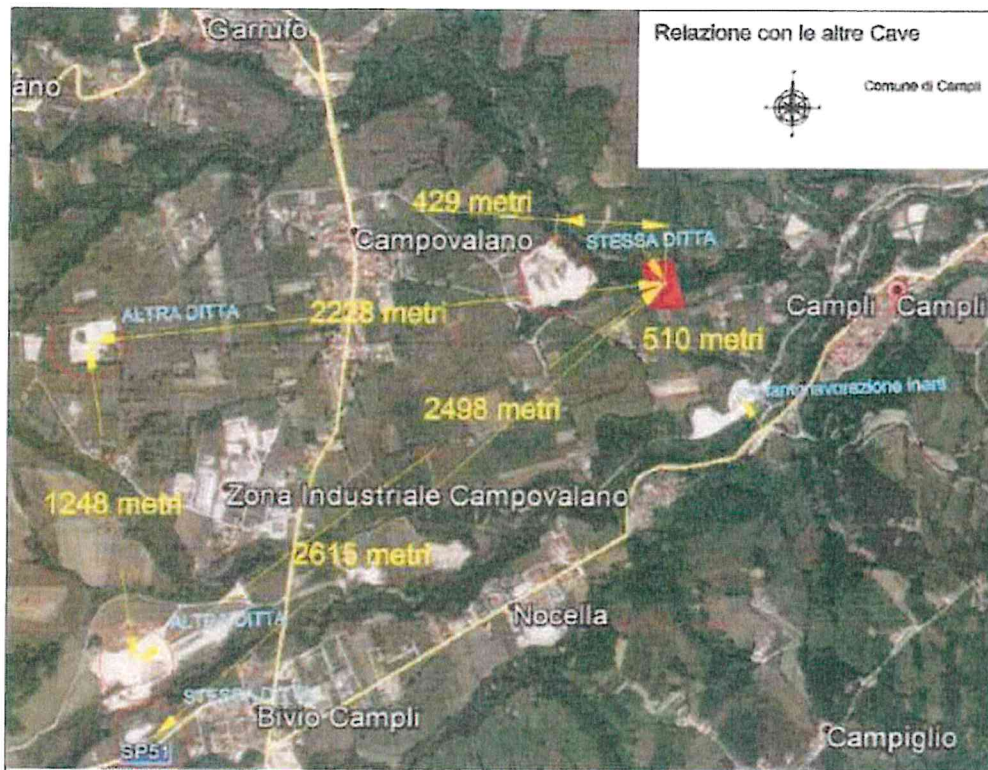
Fig. 23 - Ubicazione cave limitrofe (dallo SIA)
