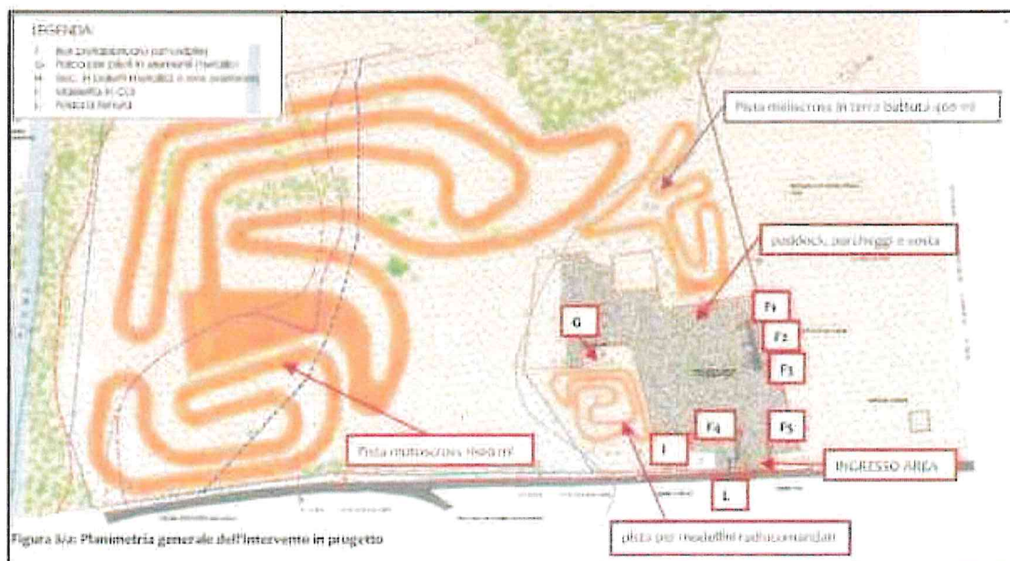
Figura 7: Planimetria generale di progetto. Le linee tratteggiate rappresentano i limiti P.S.D.A.; la linea tratteggiata in verde, in prossimità del fiume è il limite della zona SIR; la linea grigia è l'elemento di Ps segnalato nel PAI (dallo SIA).
