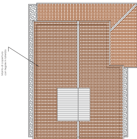
PIANTA COPERTURA
