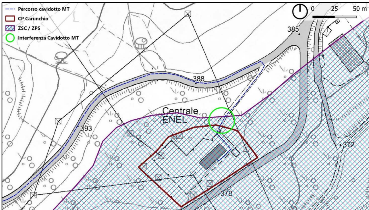
Figura 5 - Dettaglio Interferenza Cavidotto MT con ZPS / ZSC
