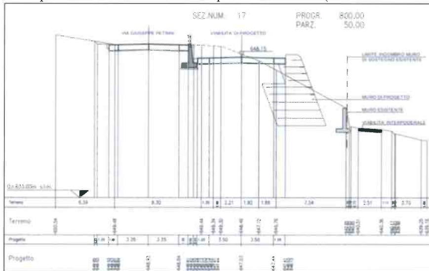
Fig. 33 – Sezione via Petri/confini zona A1 PST Colle Macchione
