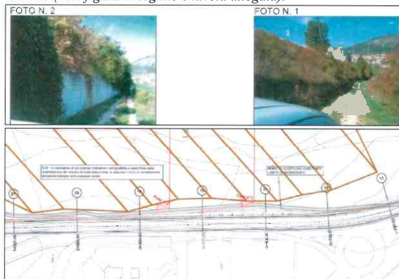
Fig. 7 – Planimetria su CTR del muro di sostegno esistente (da “QR Programmatico” allegato allo SIA)
