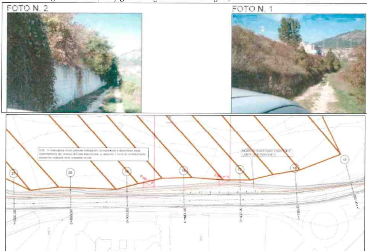
Fig. 7 – Planimetria su CTR del muro di sostegno esistente (da “QR Programmatico” allegato allo SIA)
