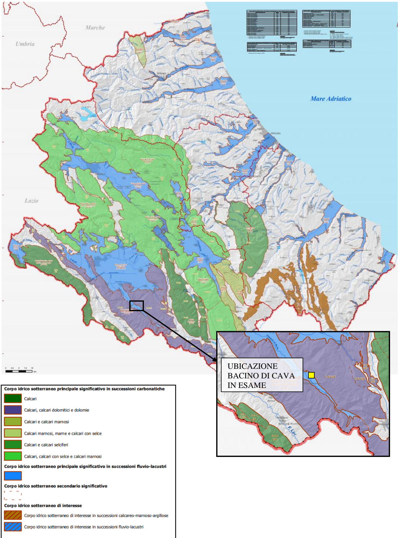
■ Stralcio Carta dei corpi idrici sotterranei significativi e di interesse ( Piano di Tutela delle Acque Regione Abruzzo )
