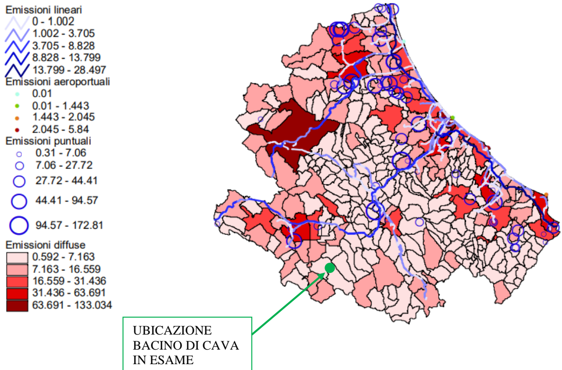
Mappa di Emissioni totali per Comune di Particelle sospese < 10 micron (PM10) [kg/anno] (Fonte Piano Regionale Tutela Qualità dell'aria – Regione Abruzzo)
