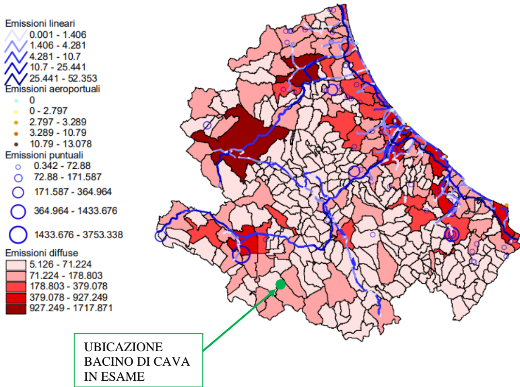
Mappa di Emissioni totali per Comune di Composti organici volatili (COV) [kg/anno] (Fonte Piano Regionale Tutela Qualità dell'aria – Regione Abruzzo)
