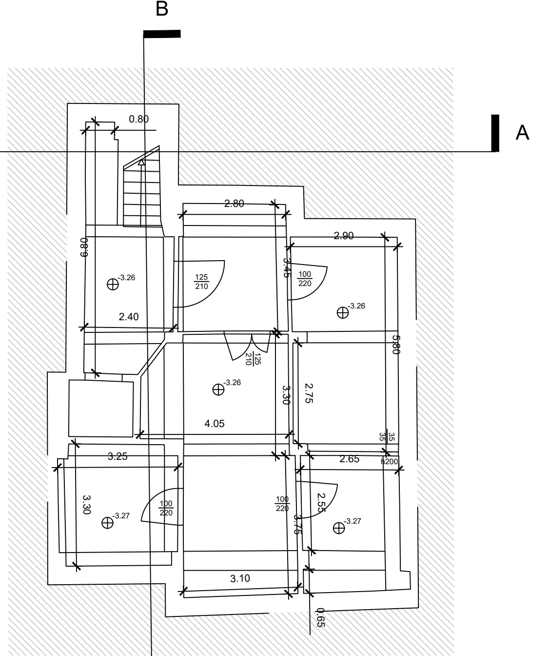
PIANTA INTERRATO
