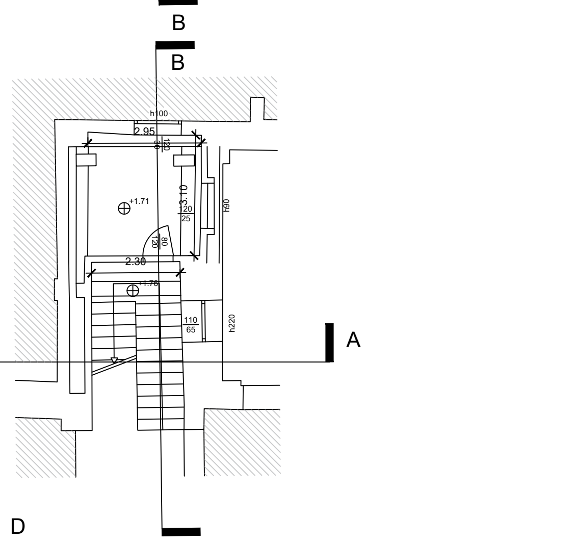
PIANTA LIVELLO +1.76
