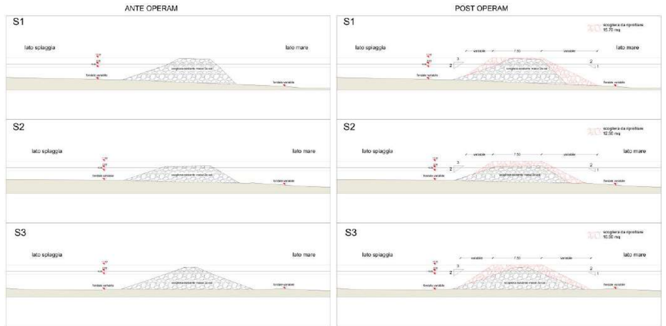
Figura 3 – Sezioni 1 – 3 della scogliera n. 7 prima e dopo l'intervento
