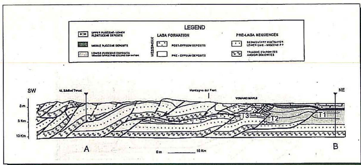
Fig.2: sezione del sistema a thrust marchigiano abruzzese
