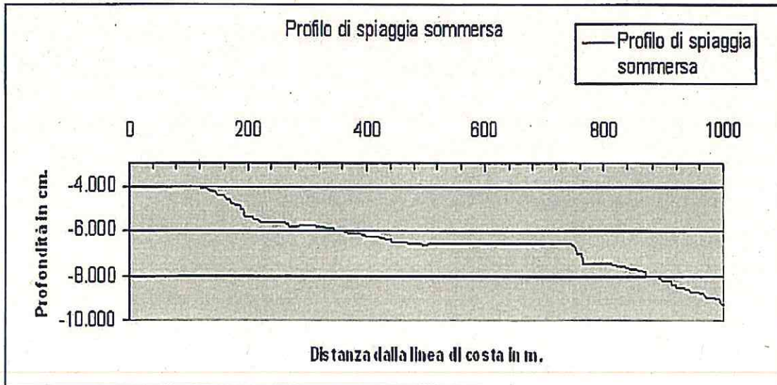
Fig 17: profilo di spiaggia sommersa
