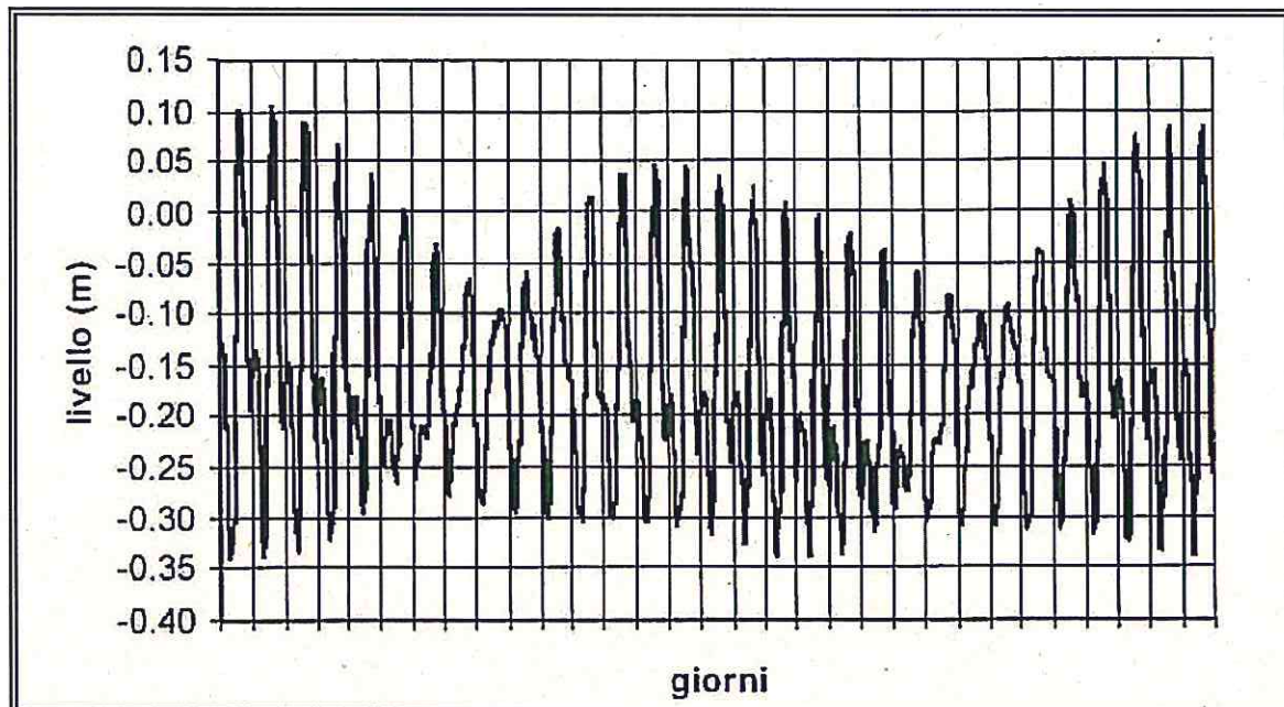
Fig 8: ricostruzione onda di marea.
