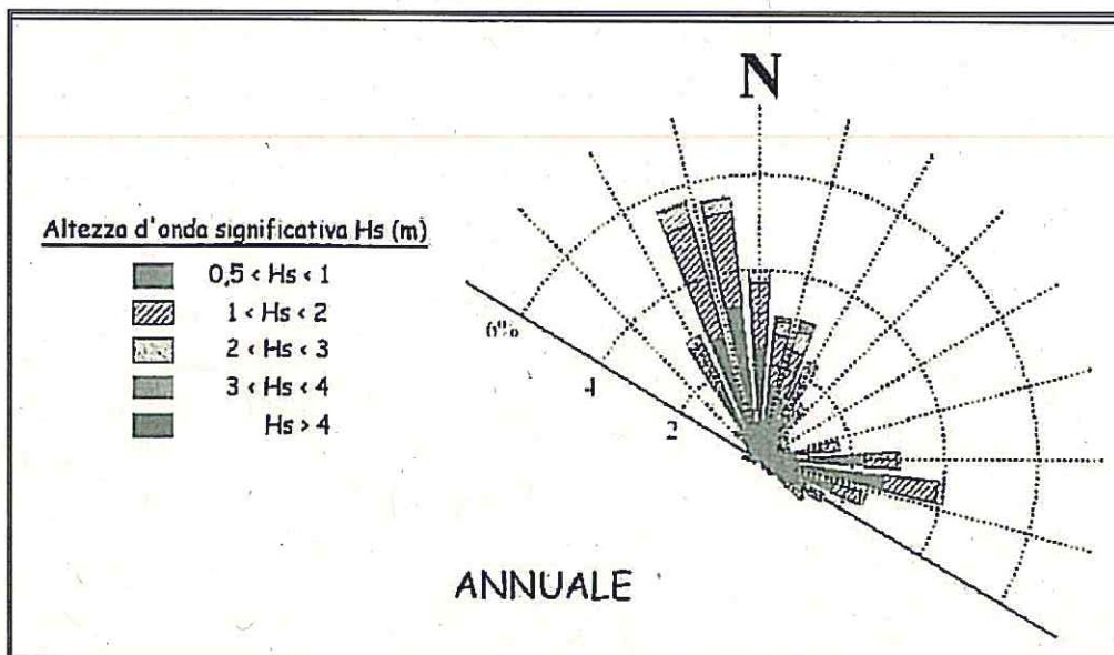
Fig 14: direzione del moto ondoso
