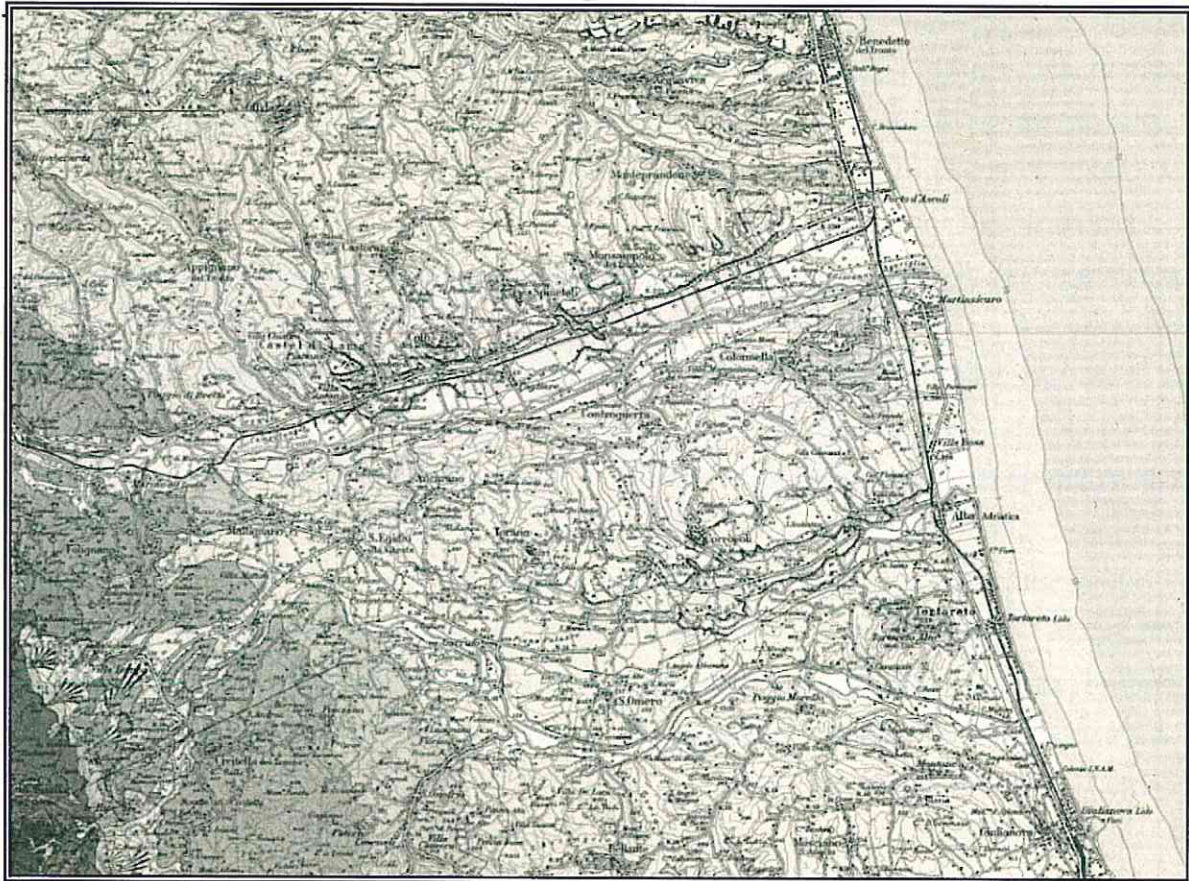
Fig.4 carta geologica con indicati in azzurro bacini idrografici
