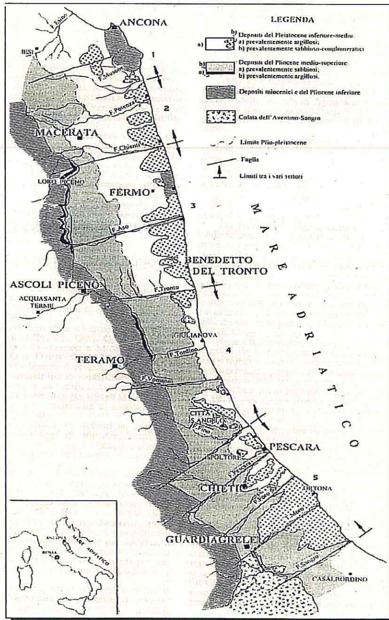
Fig.3:carta geologica schematica del bacino periadriatico
