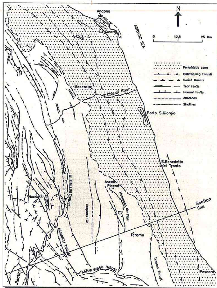
Fig.1: schema strutturale del sistema a thrust marchigiano abruzzese
