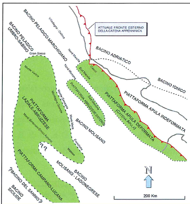
Fig. 2: Ricostruzione della distribuzione paleogeografica delle principali unità di piattaforma e di bacino coinvolte nella struttura della catena centro apenninica (Vezzani et alii. 2004)
