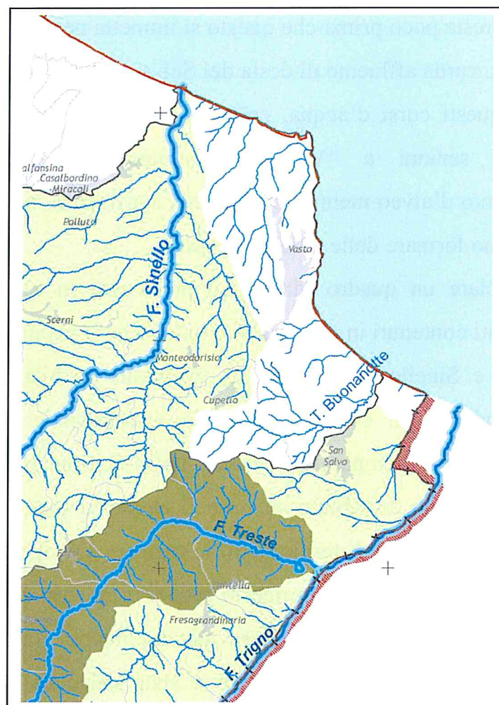
Fig. 6: La rete idrografica nell'area in esame (da Regione Abruzzo, Piano di Tutela delle Acque)
