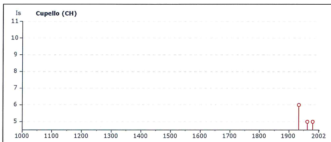
Fig. 10: Storia sismica del comune di Cupello dal 1000 al 2002. Sulle ordinate sono riportate le intensità sismiche (Is) e sulle ascisse il riferimento temporale espresso in anni
