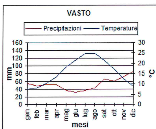
Fig. 7: Rapporto precipitazioni-temperature registrate nella stazione pluviotermometrica di Vasto
