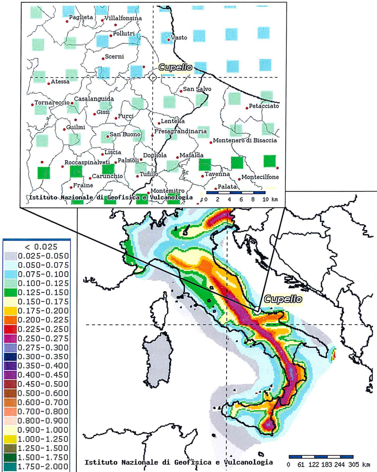
Fig.12: Mappa di pericolosità sismica espressa in termini di accelerazione massima del suolo con probabilità di eccedenza del 10% in 50 anni riferita a suoli rigidi ( V_{s30} > 800 m/s) (da Istituto Nazionale di Geofisica e Vulcanologia).
