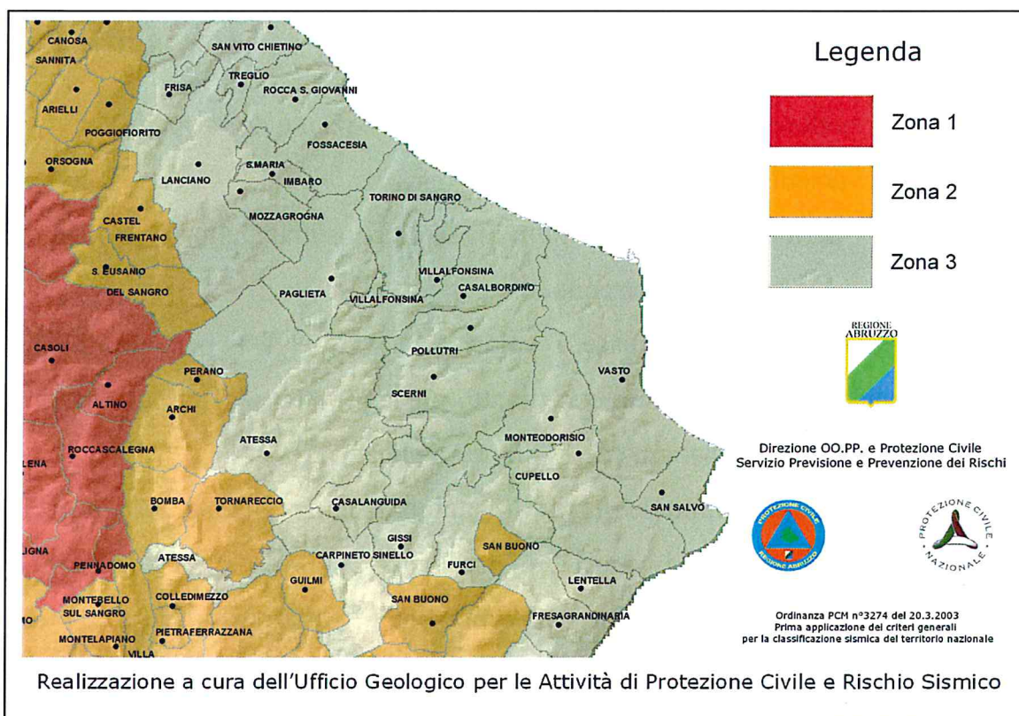
Fig. 11: Mapa sismica regionale
