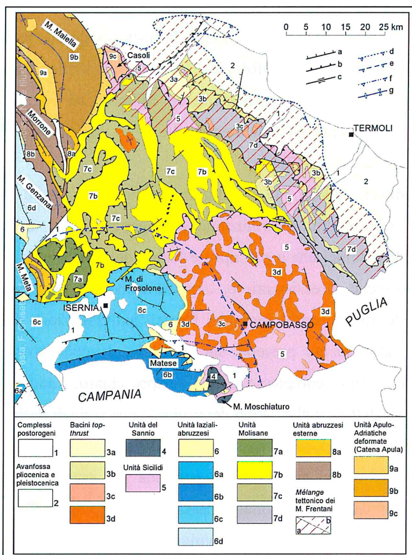
Fig. 4: Schema geologico-strutturale dell'Appennino abruzzese-molisano
