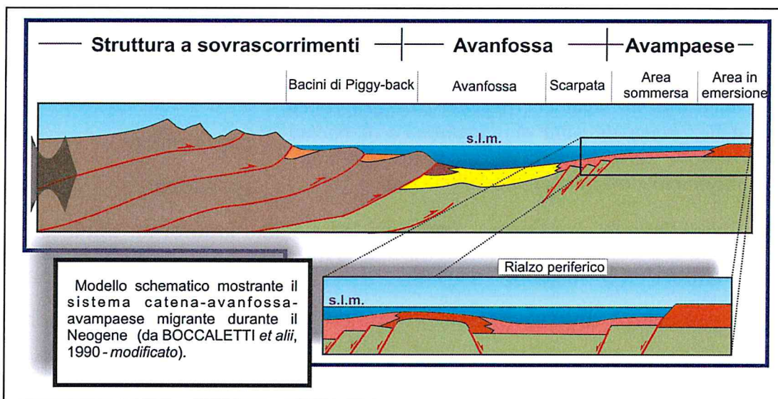
Fig. 3: Schema del sistema catena-avanfossa-avampaese
