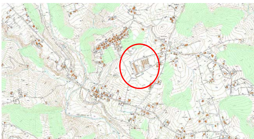
Figura 4: Stralcio Carta del Rischio - Assetto Idrogeologico PAI Regione Abruzzo.
