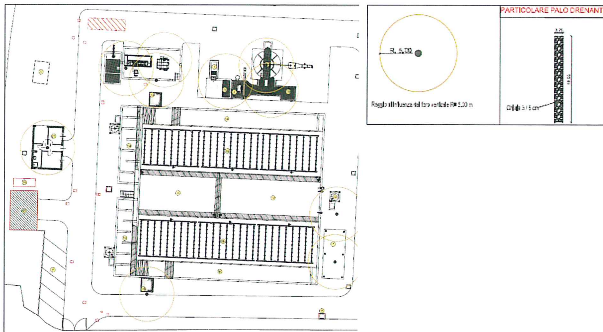
Fig. 9 – Ubicazione pali drenanti (da Elaborati integrativi allo SPA)
