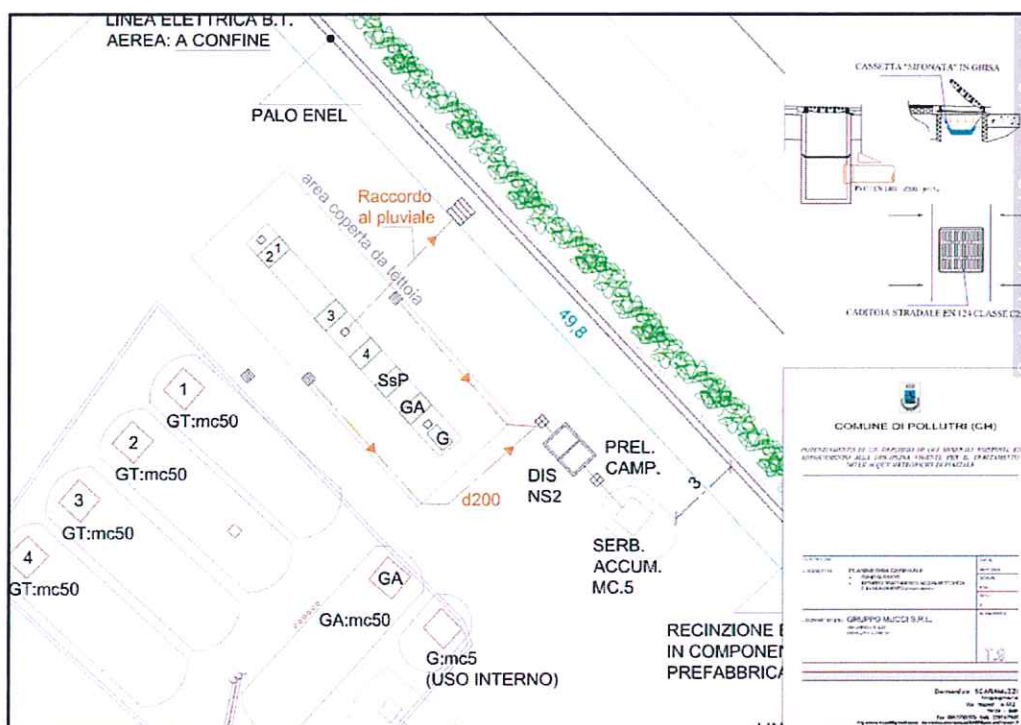
Figura 3: Planimetria impianto trattamento acqua meteorica e dilavamento (da allegato P2_B alle integrazioni).
