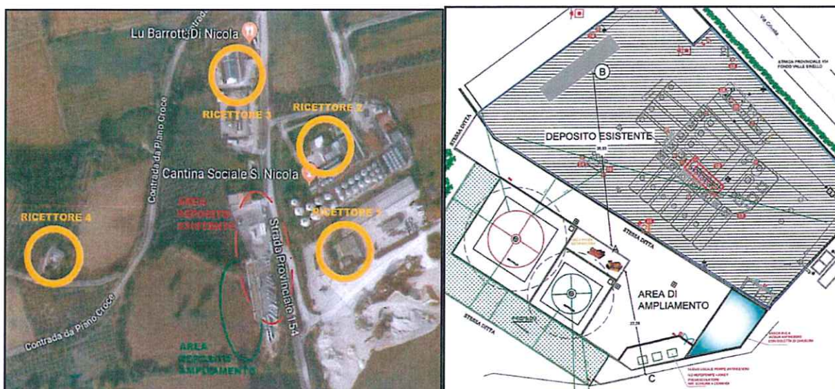
Figura 1: Planimetria recettori (a destra) e punti di misura (a sinistra) (da allegato P1 alle integrazioni).
