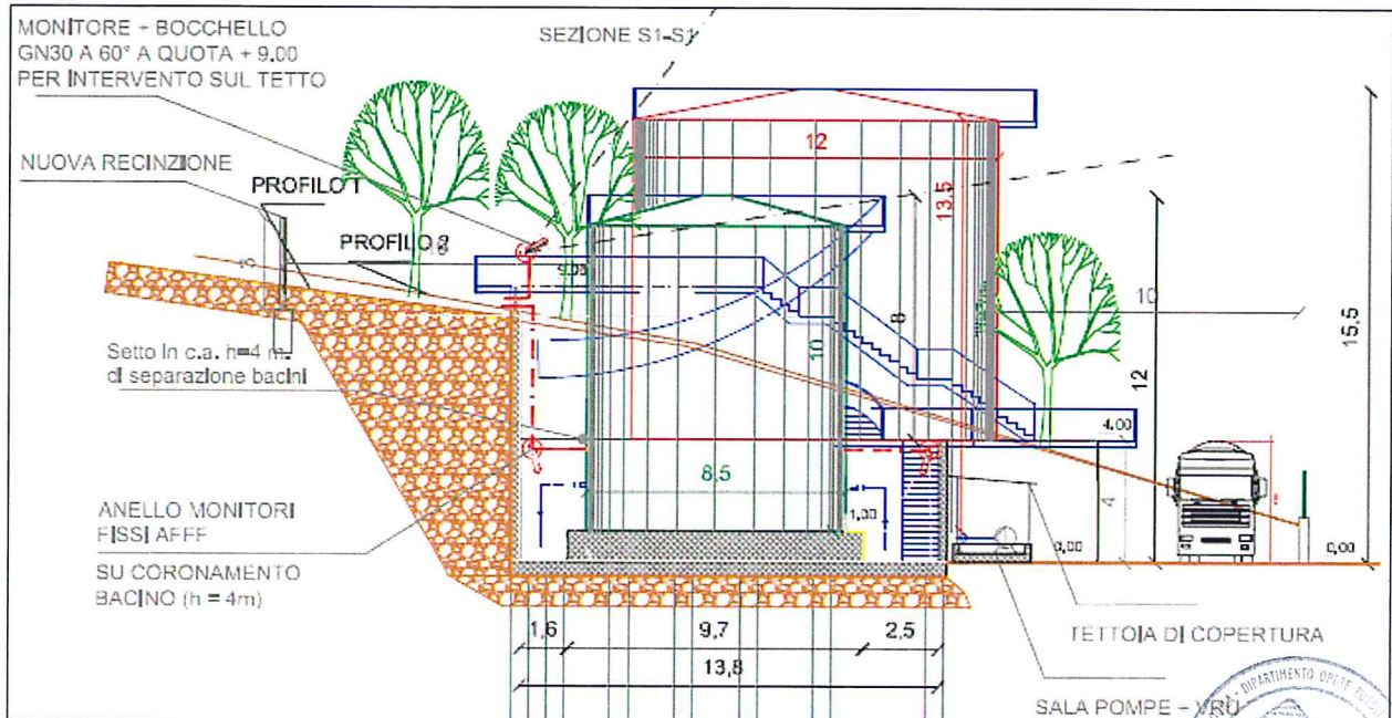
Fig. 13a - Sezioni di progetto (da Elab. T9 allegato allo SPA)
