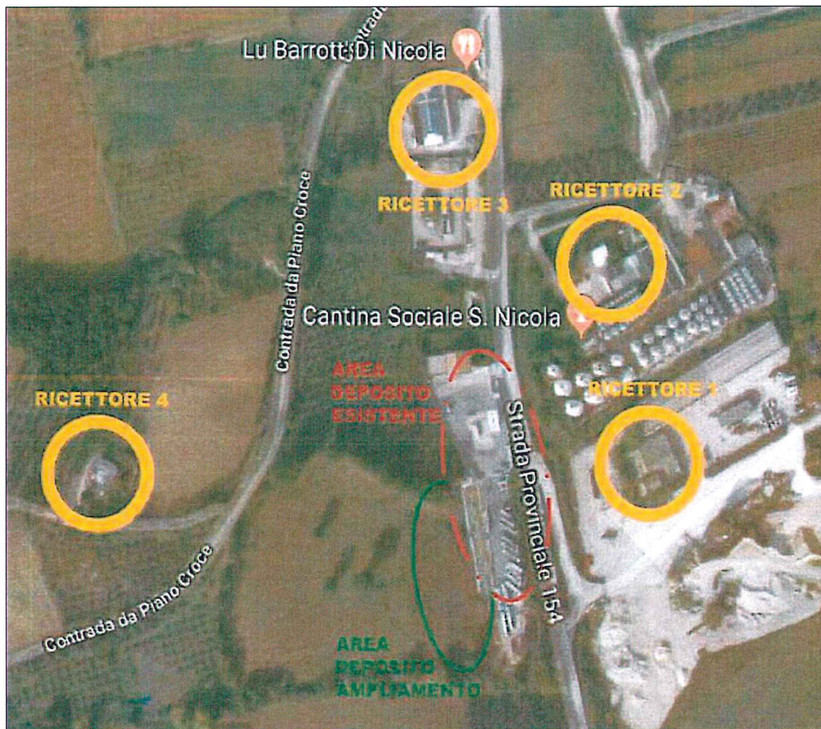
Fig. 5 – Planimetria recettori (da Elab. P4 integrato allo SPA)
