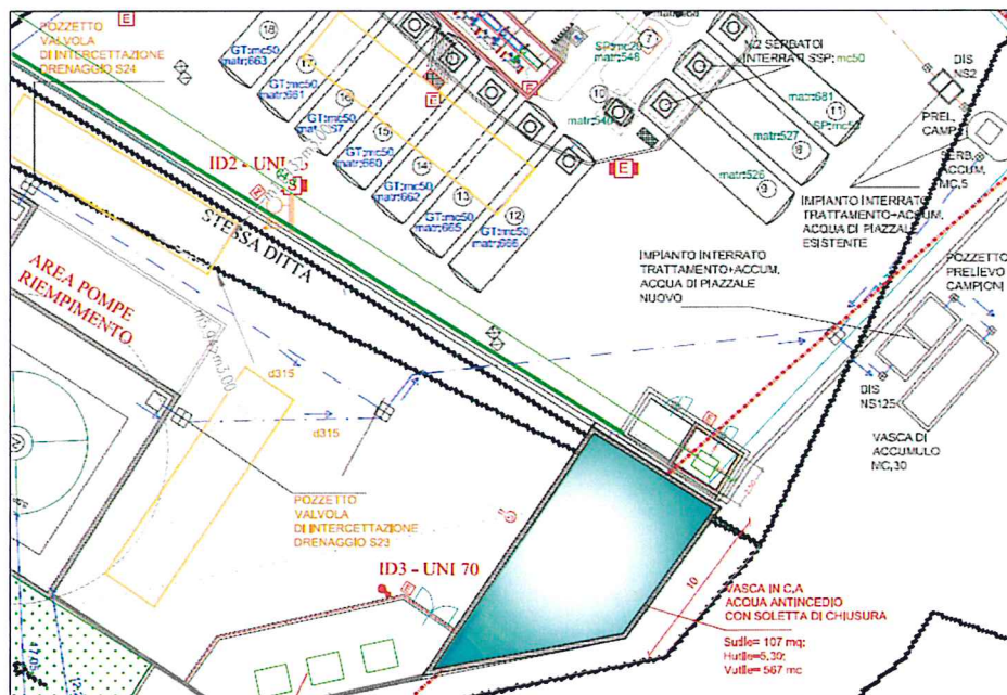
Fig. 18 – Impianto di drenaggio e trattamento acque di piazzale (da Elab. T7 allegato allo SPA)
