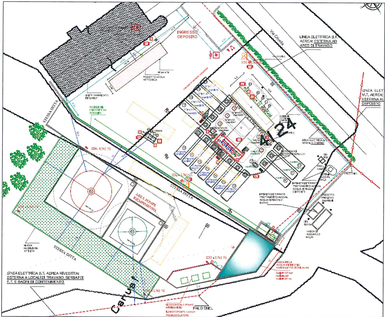
Fig. 12 - Planimetria di progetto (da Elab. T5 allegato allo SPA)
