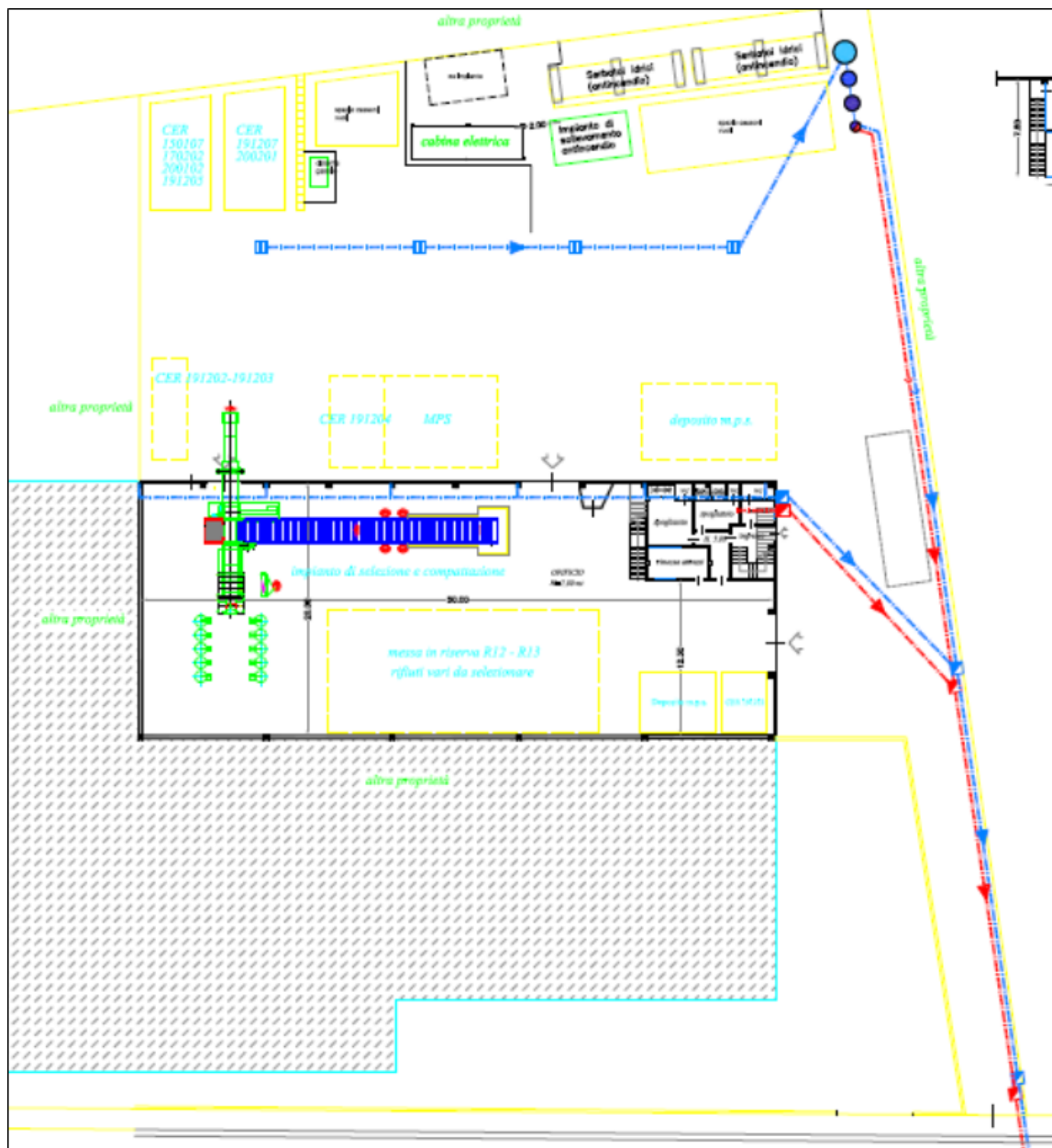
Layout impianto (da Elab. "Allegati" allegato allo SPA)
