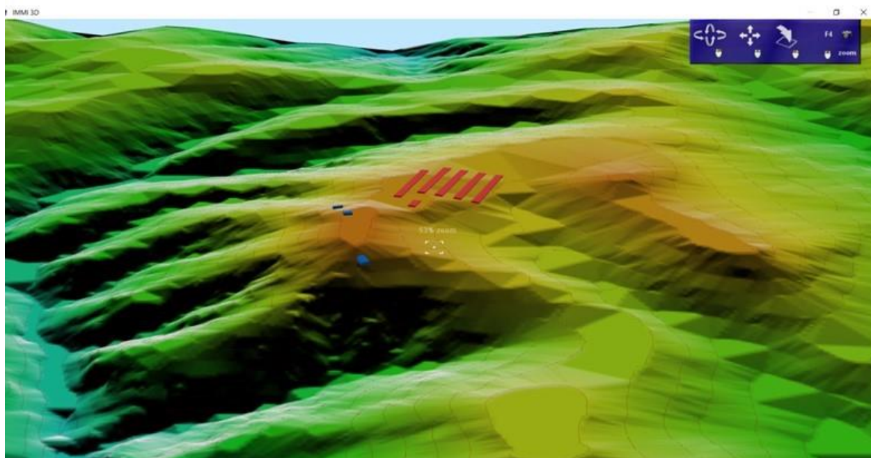
Figura 6 – Modellizzazione 3D del terreno con posizione dei capannoni da software IMMI
