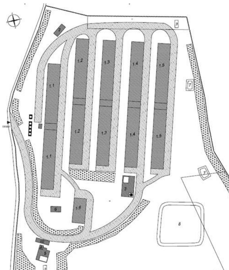
Figura 3 – Planimetria Allevamento avicolo Pozzo Notaresco
