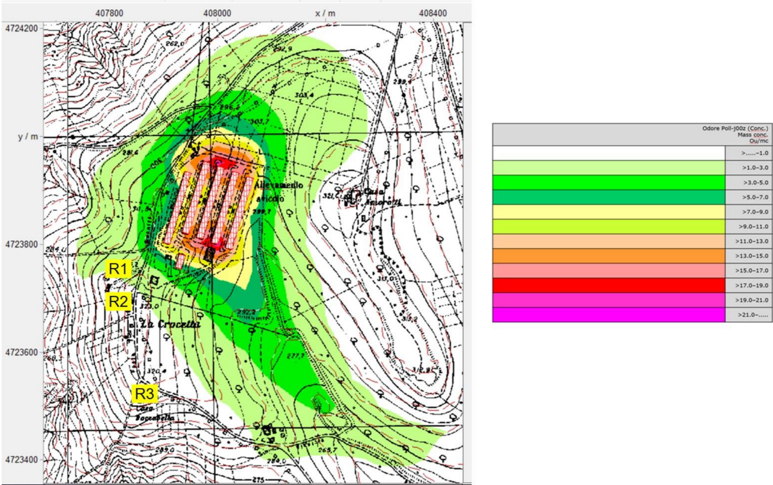
Figura 20 - Simulazione dispersione sostanze odorigene - Fattore medio da documento BREF 2017 - Tabella 3.53
