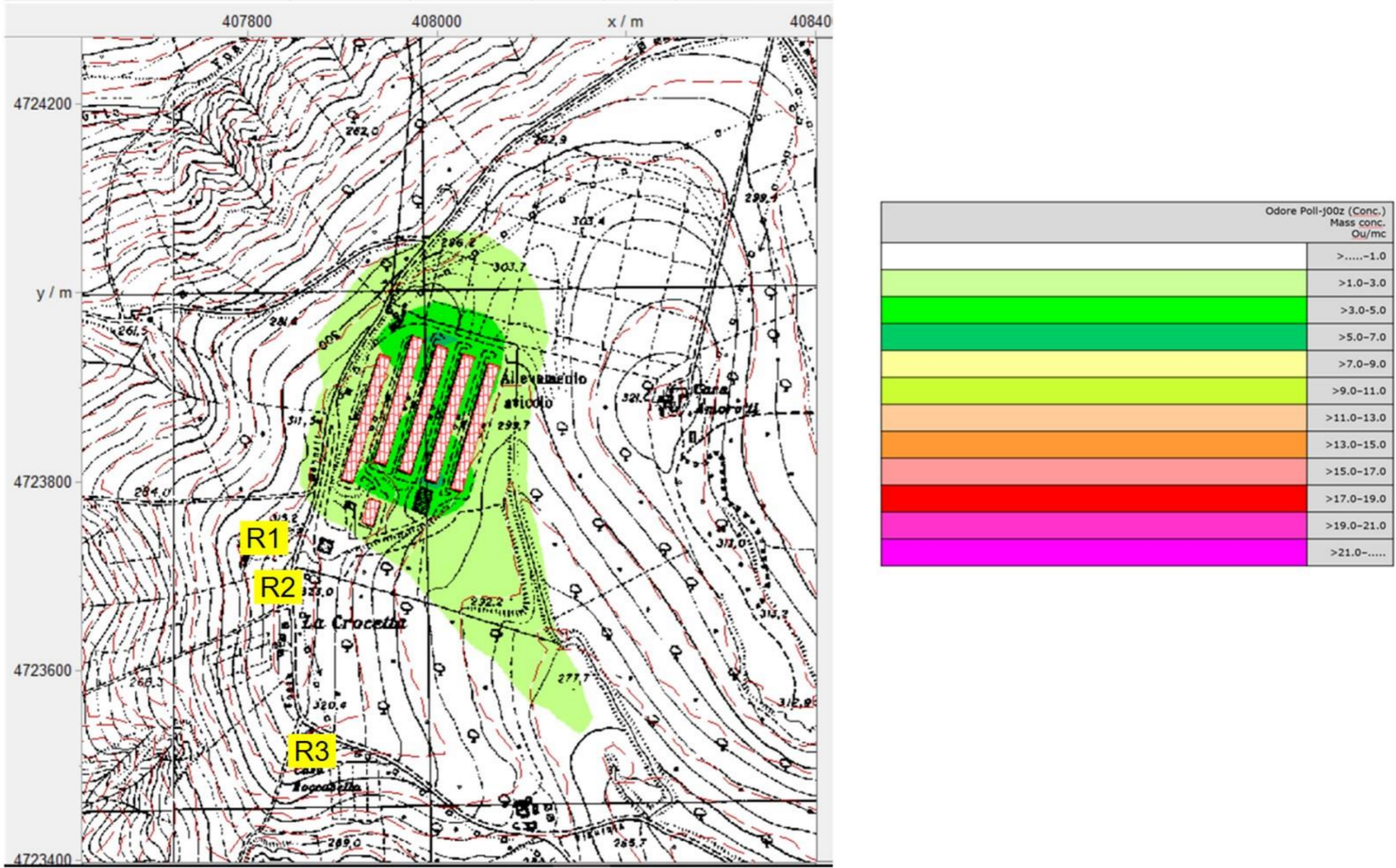
Figura 21 – Simulazione dispersione sostanze odorigene – Fattore da documento BREF 2017 – Tabella 4.55
