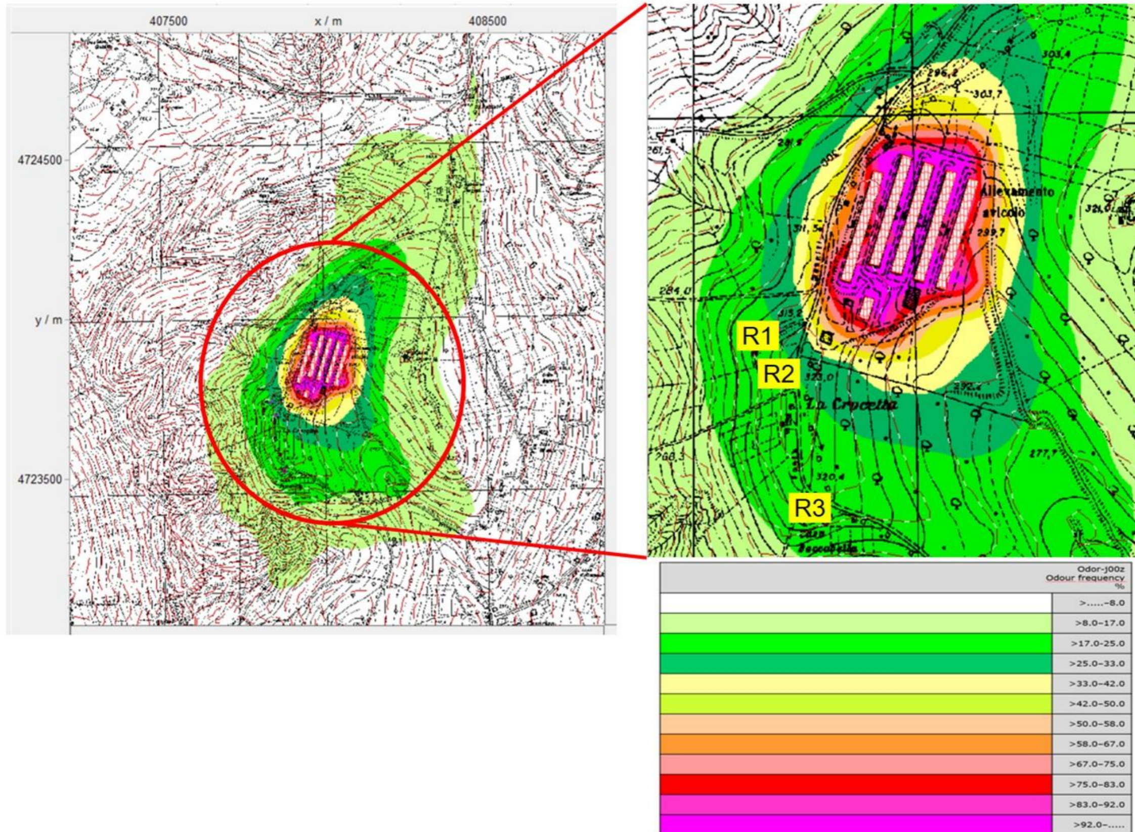
Figura 16 - Simulazione dispersione sostanze odorigene - Fattore massimo da documento BREF 2017 - Tabella 3.53
