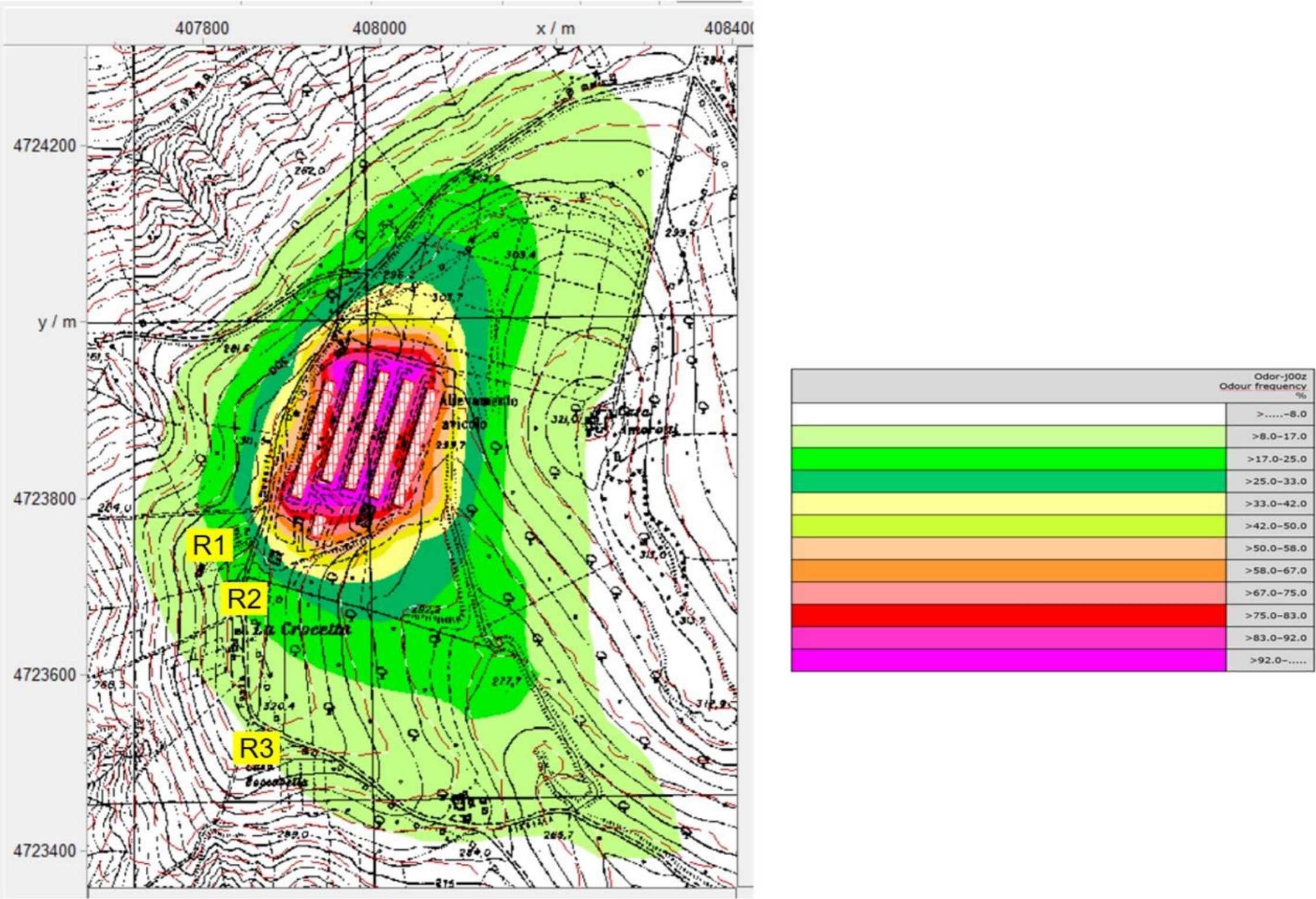
Figura 18 – Simulazione dispersione sostanze odorigene – Fattore da documento BREF 2017 – Tabella 4.55
