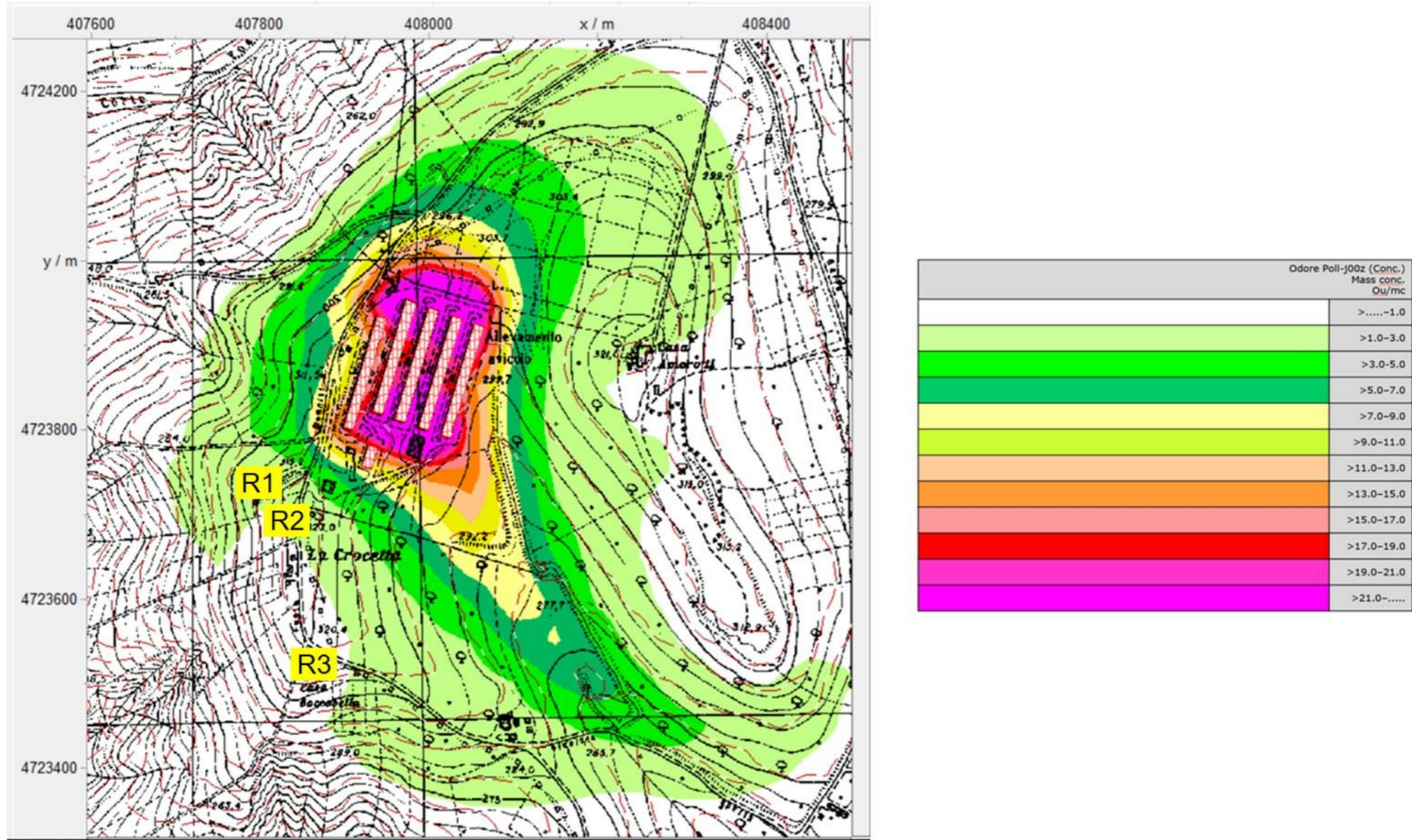
Figura 19 – Simulazione dispersione sostanze odorigene – Fattore massimo da documento BREF 2017 – Tabella 3.53
