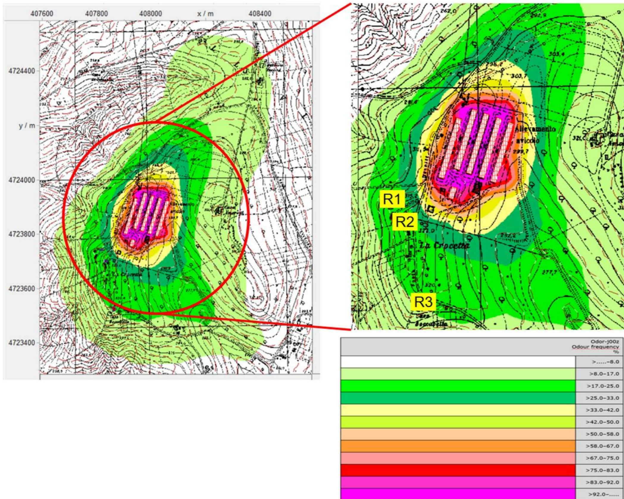
Figura 17 – Simulazione dispersione sostanze odorigene – Fattore medio da documento BREF 2017 – Tabella 3.53
