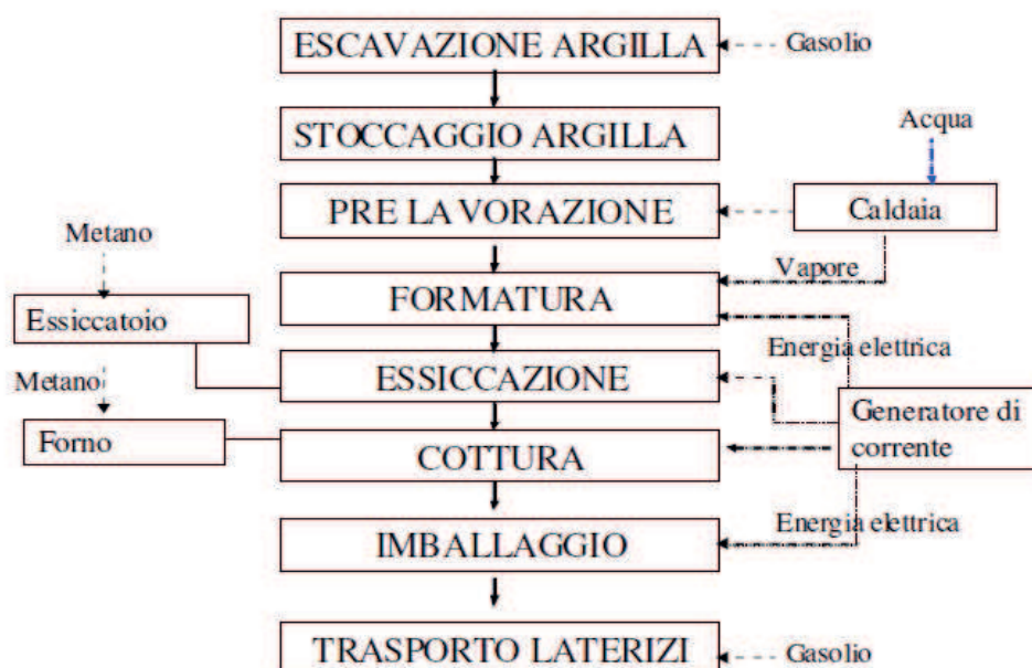
Fig. 16. Schema flusso ciclo produttivo
