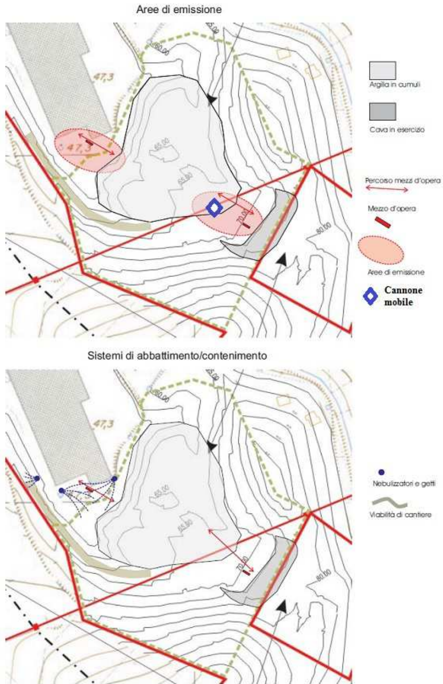
Fig. 37. Area di interesse con indicati sistemi abbattimento emissioni polverulente
