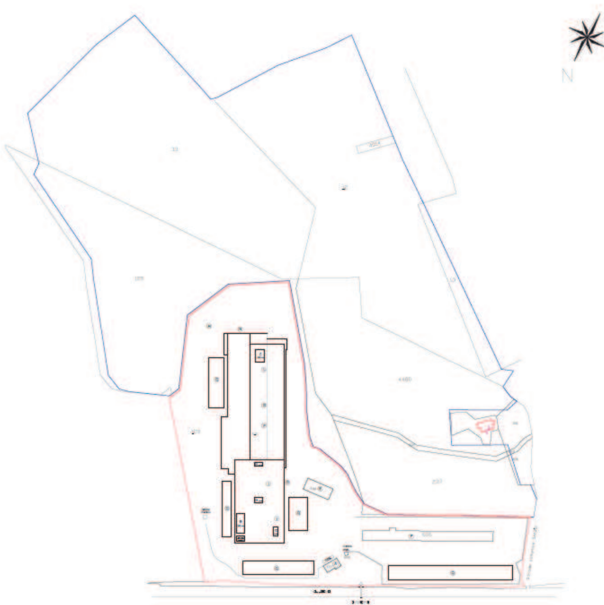
Fig. 15. Planimetria generale sito. Perimetrata in rosso area produzione laterizi e recupero rifiuti non pericolosi - perimetrata in blu area di cava
