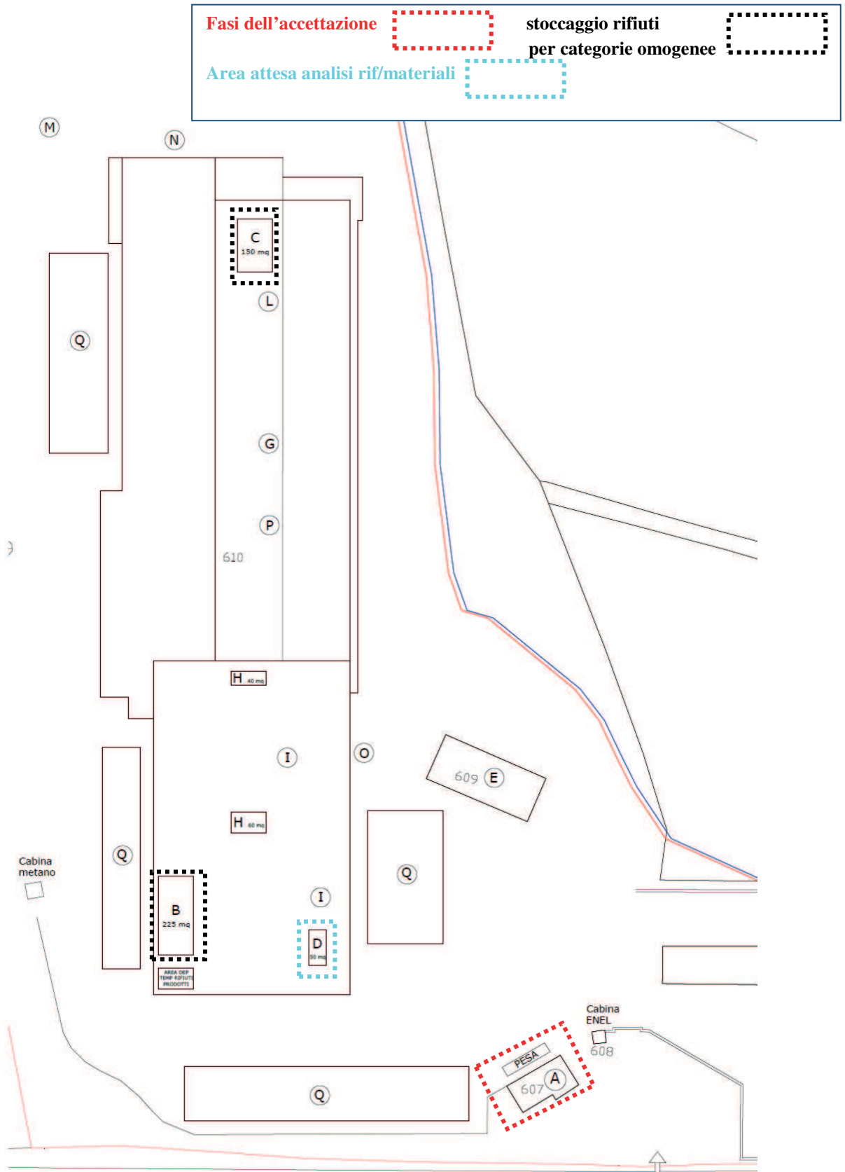
Fig. 17. Aree accettazione e scarico dei rifiuti
