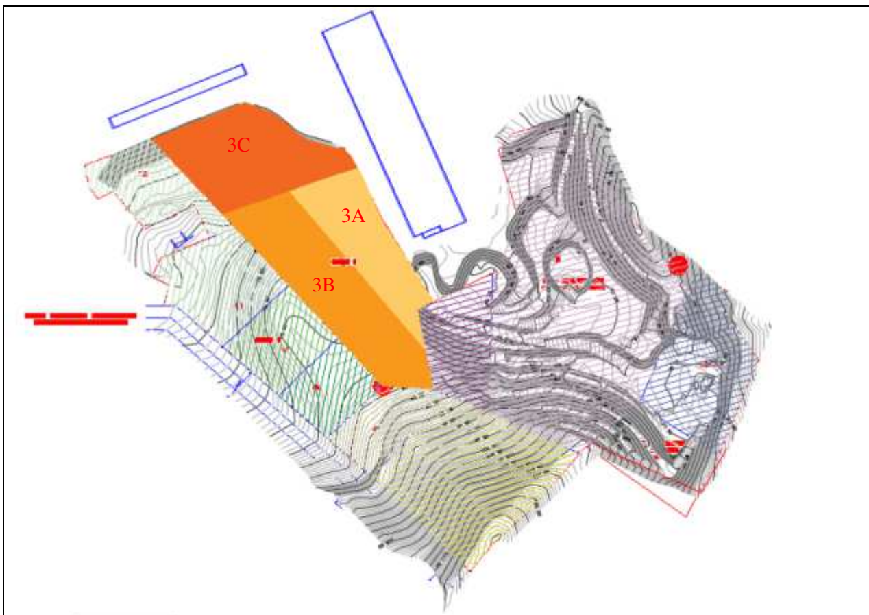
Fig. 32. Planimetria di progetto Lotto 3
