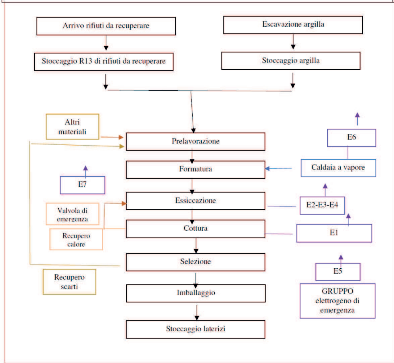
Fig. 19. Schema di flusso con rifiuti
