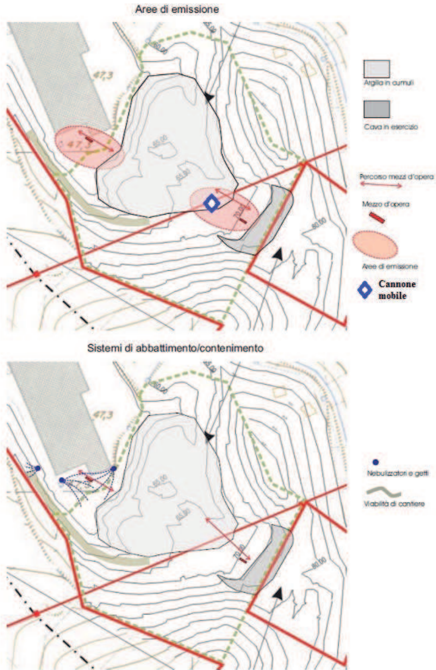
Fig. 20. Area di interesse con indicati sistemi abbattimento emissioni polverulente
