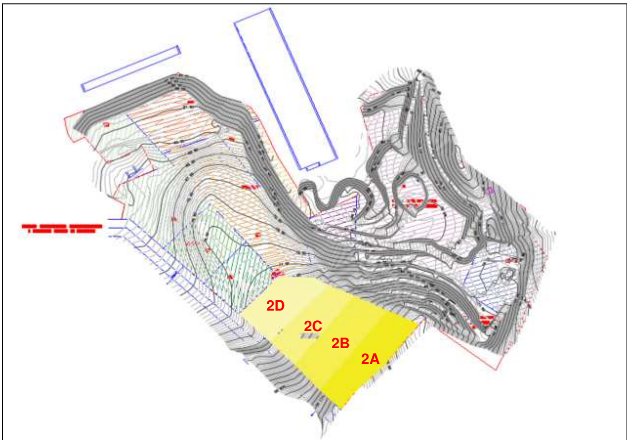
Fig. 31. Planimetria di progetto Lotto 2
