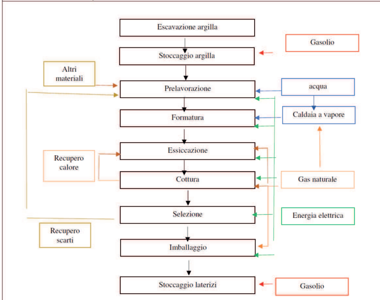
Fig. 18. Schema di flusso attuale
