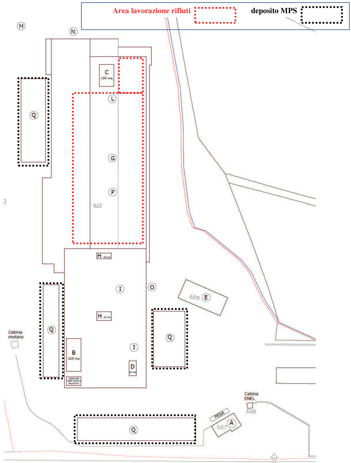
Fig. 21. Area lavorazione rifiuti e deposito MPS
