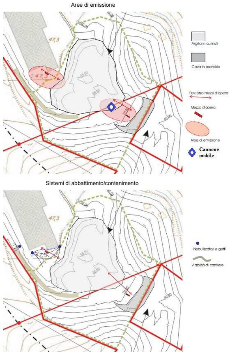
Fig. 43. Area di interesse con indicati sistemi abbattimento emissioni polverulente
