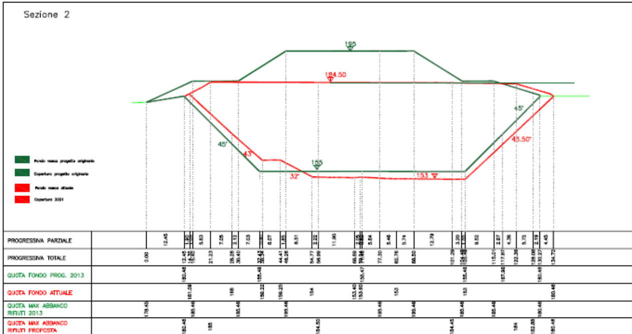
Fig. 2: sezione trasversale - lotto 2
