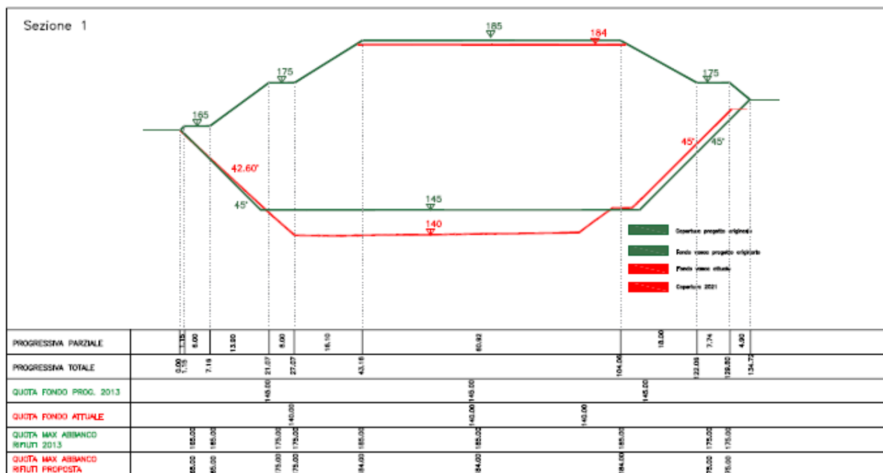
Fig. 1: sezione trasversale - lotto 1
