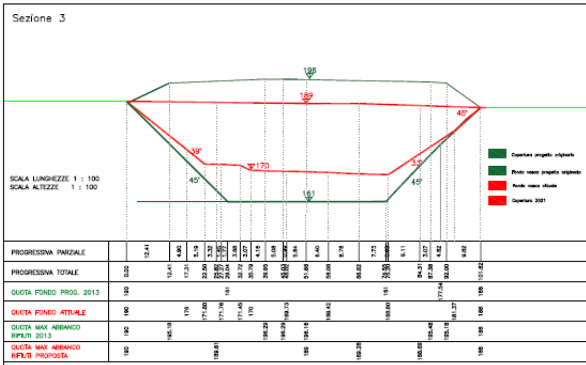
Fig. 3: sezione trasversale - lotto 3
