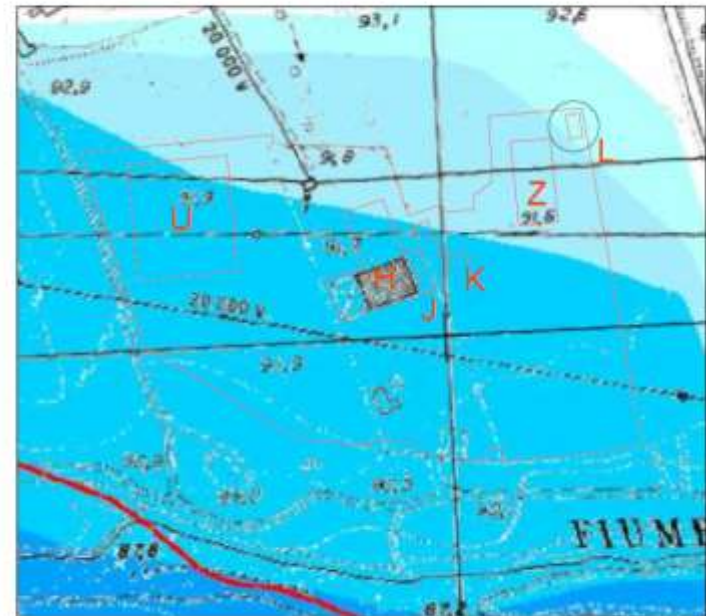
STATO MODIFICATO
