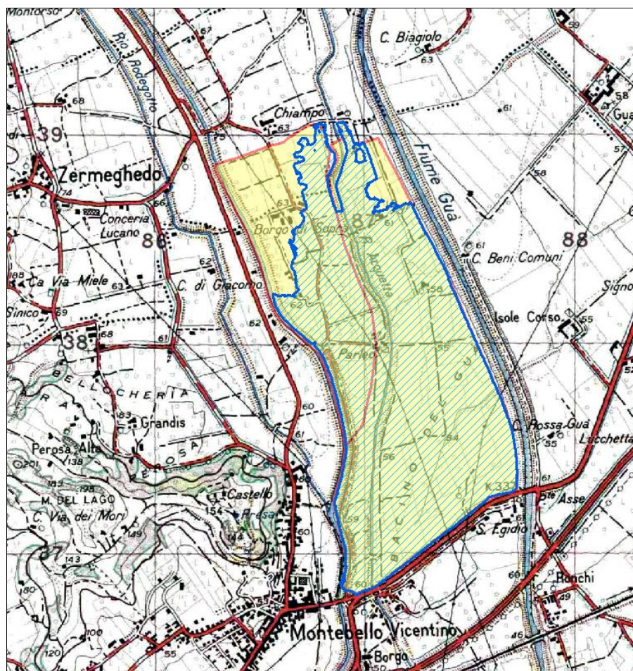
Figura 1.3 – Area di intervento (in giallo è indicata l'area destinata al bacino nello stato di progetto, con il retino blu è indicata l'area attuale di invaso).
