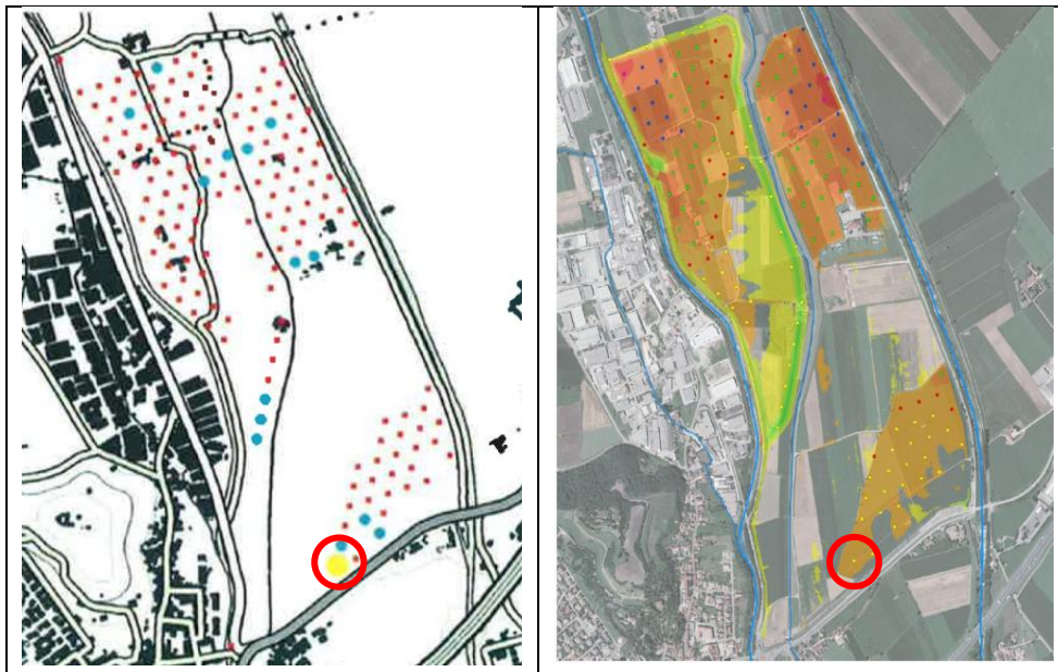
Figura 2.1 – Planimetria posizione indagini ambientali PD (cerchiato in rosso il sondaggio S154 con superamento del limite di colonna B
