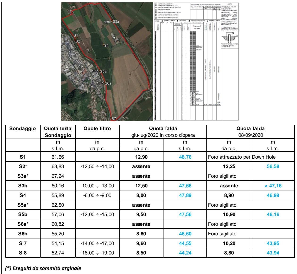
Figura 1.13 – Ubicazione dei sondaggi a carotaggio continuo attrezzati con piezometri Casagrande e livelli piezometrici misurati.
