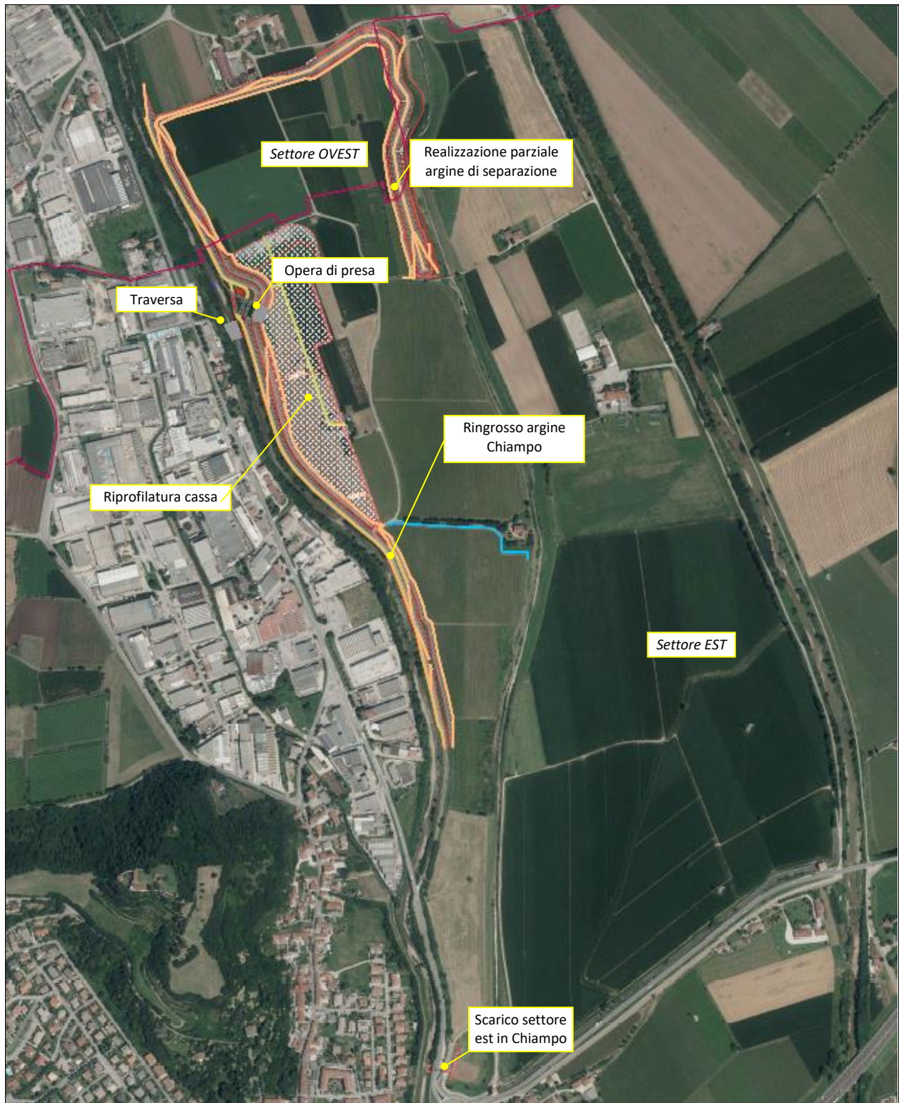
Figura 1.6 – Planimetria con indicazione degli interventi di progetto – primo stralcio funzionale..
