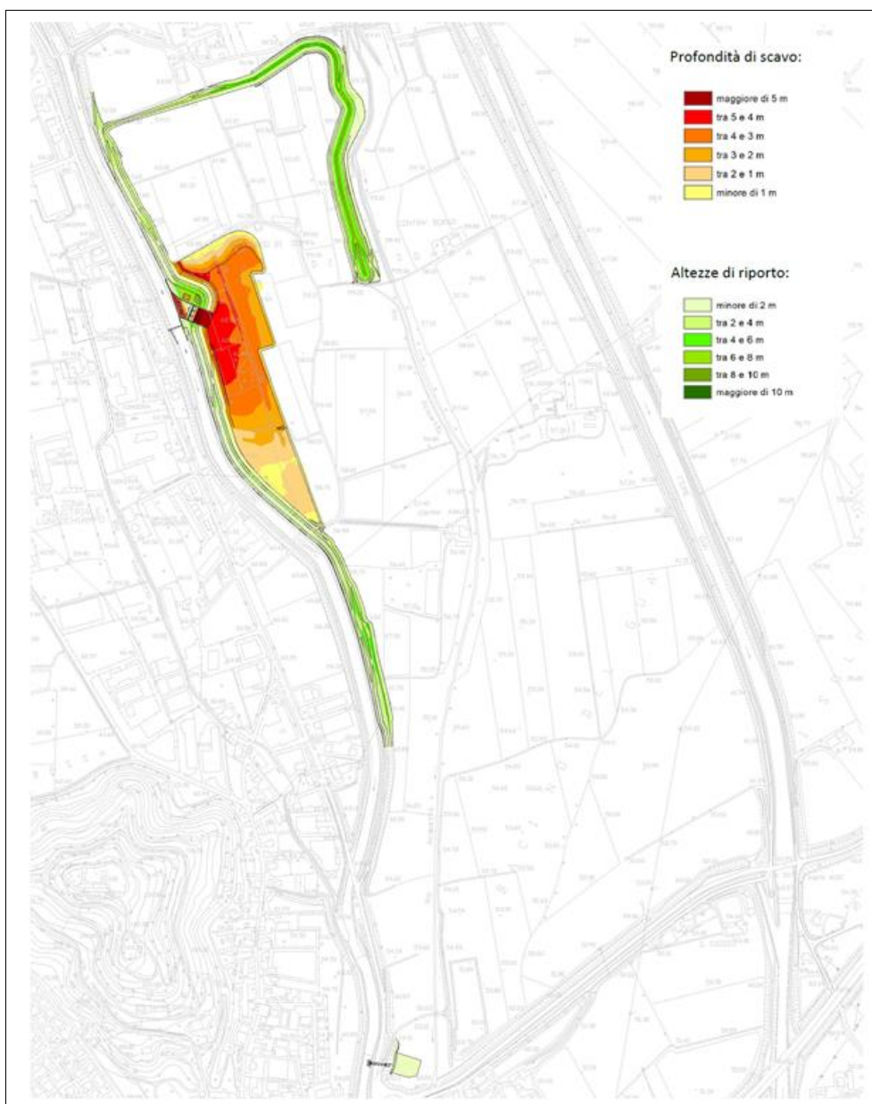
Figura 1.7 – Ubicazione delle opere con indicazione delle aree di scavo (nei toni di giallo-rosso) e riporto (nei toni di verde).
