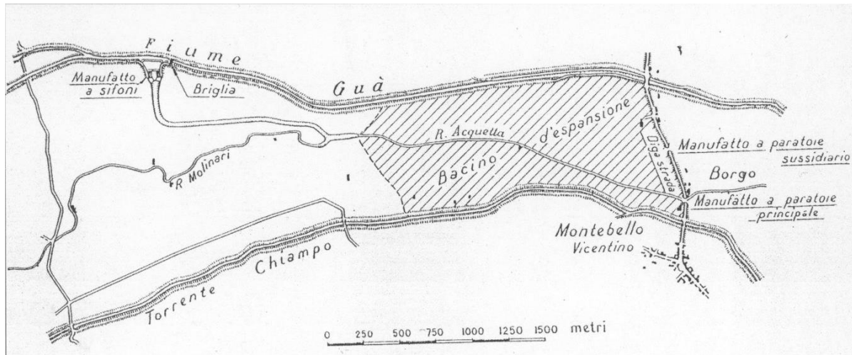
Figura 1.4 - Planimetria del bacino idraulico di Montebello (da Miliani, 1939).
