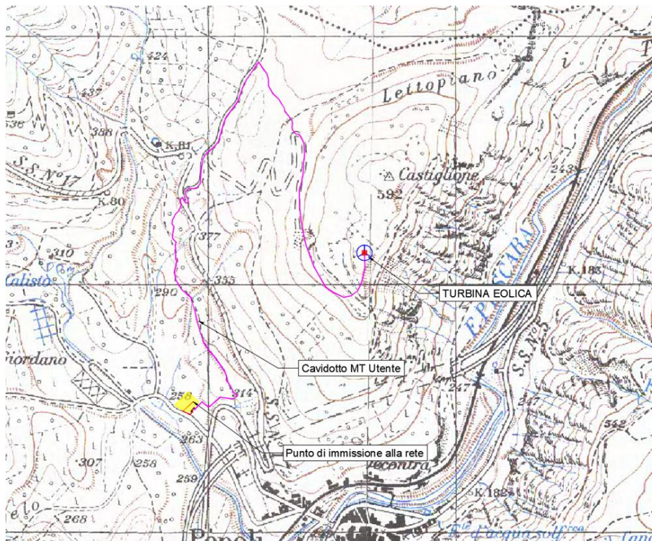
Inquadramento dell'area d'impianto e delle opere connessione su carta IGM
