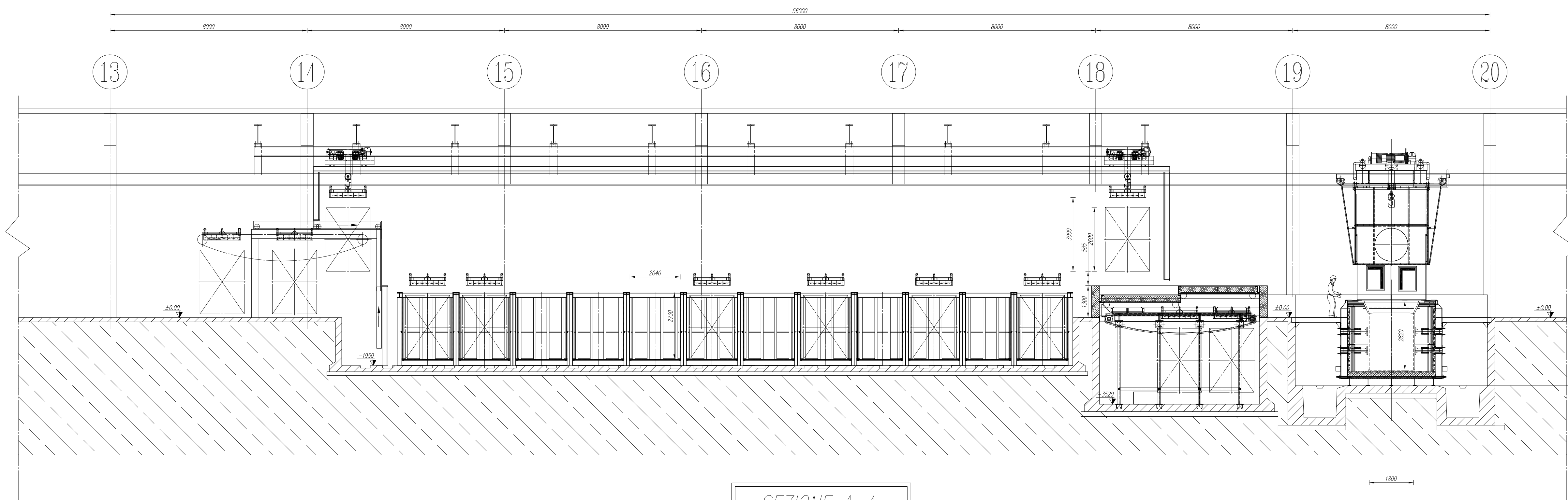
SEZIONE A-A SCALA 1:150
