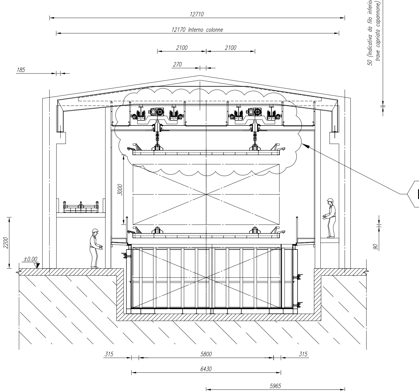
SEZIONE C-C SCALA 1:150
